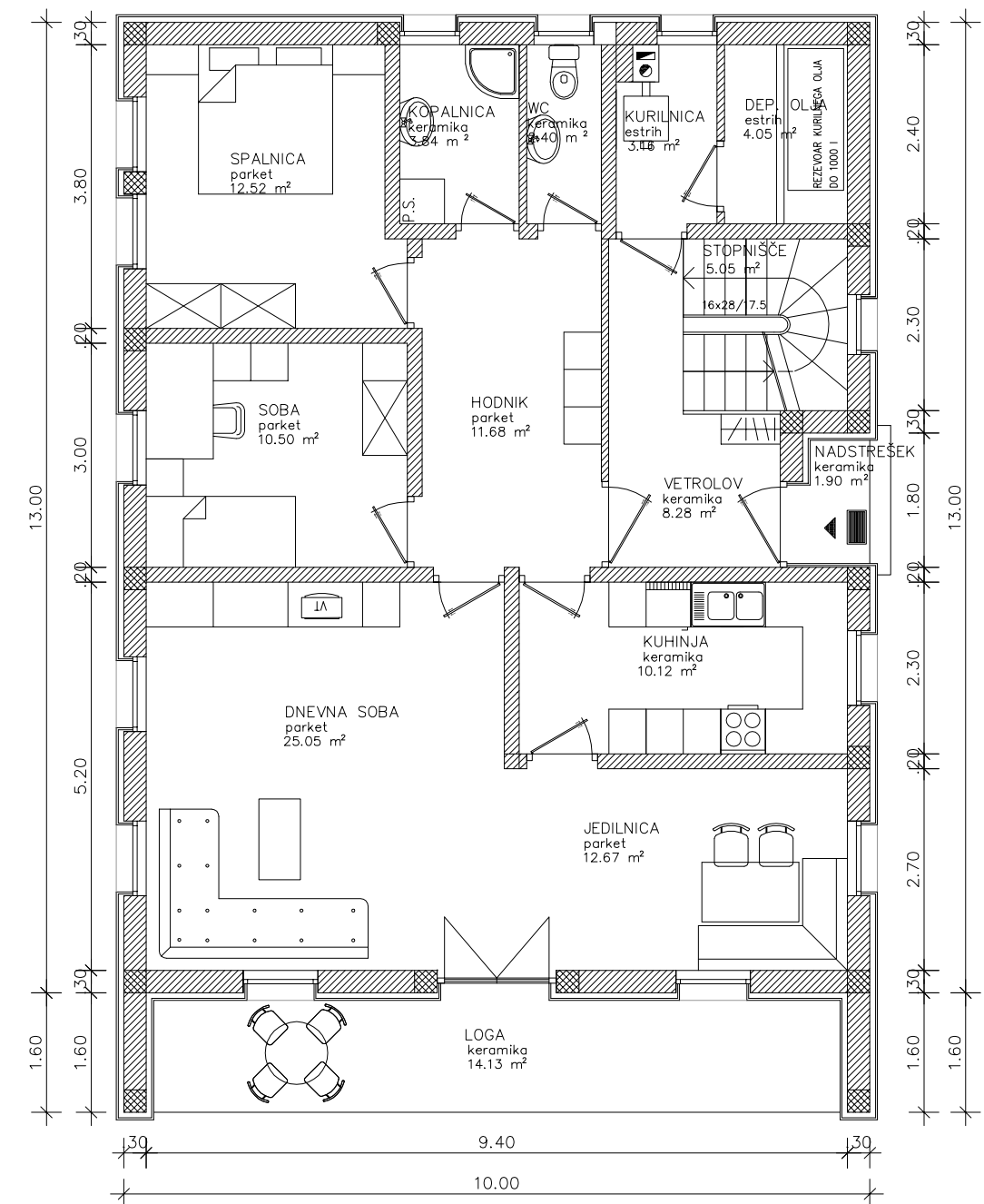
10.00 1.30 3.20 2.00 1.60 1.00 2.00 1.35 1.65 1.30 TLORIS PRITLIČJA
