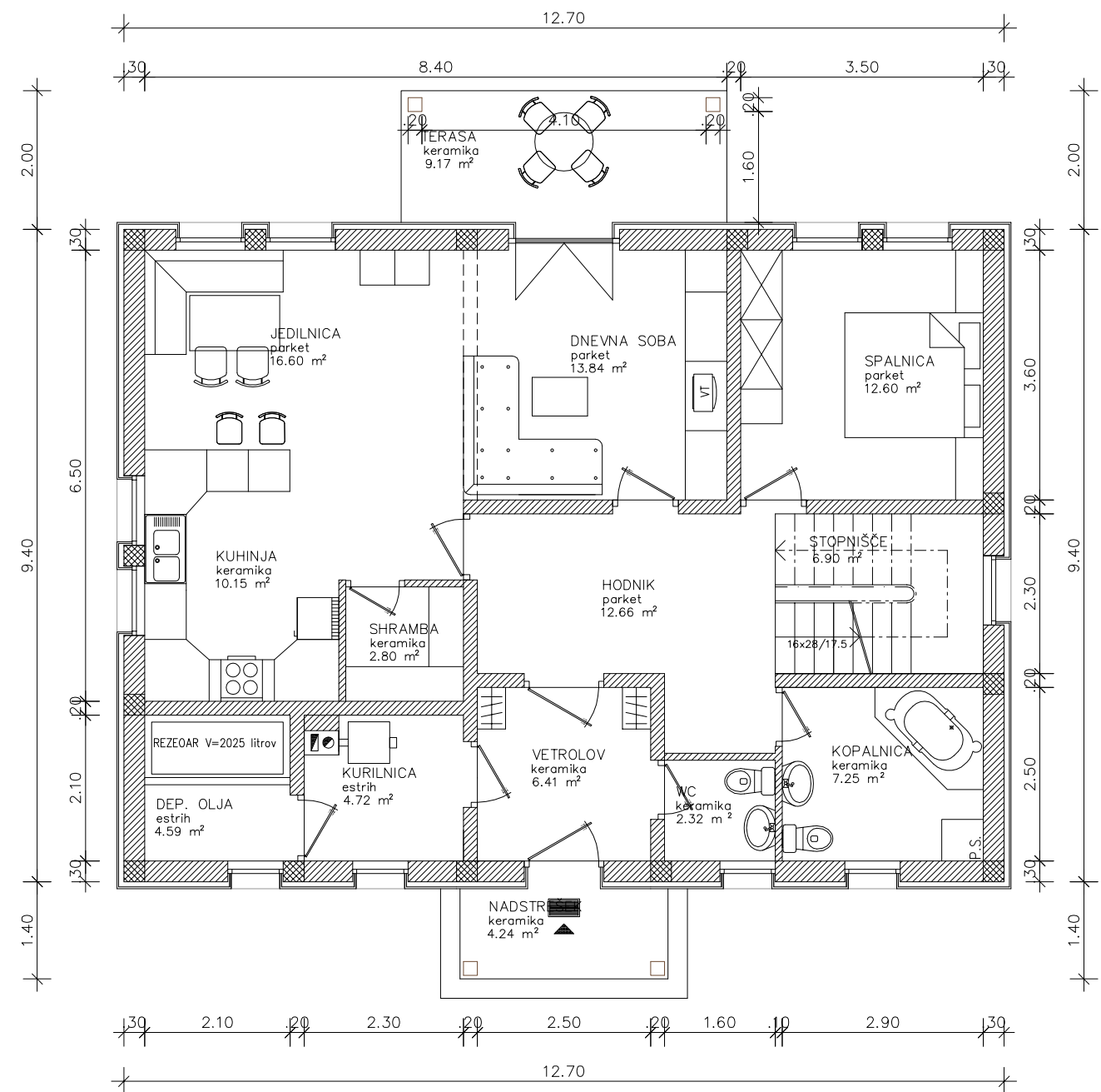
TLORIS PRITLIČJA
