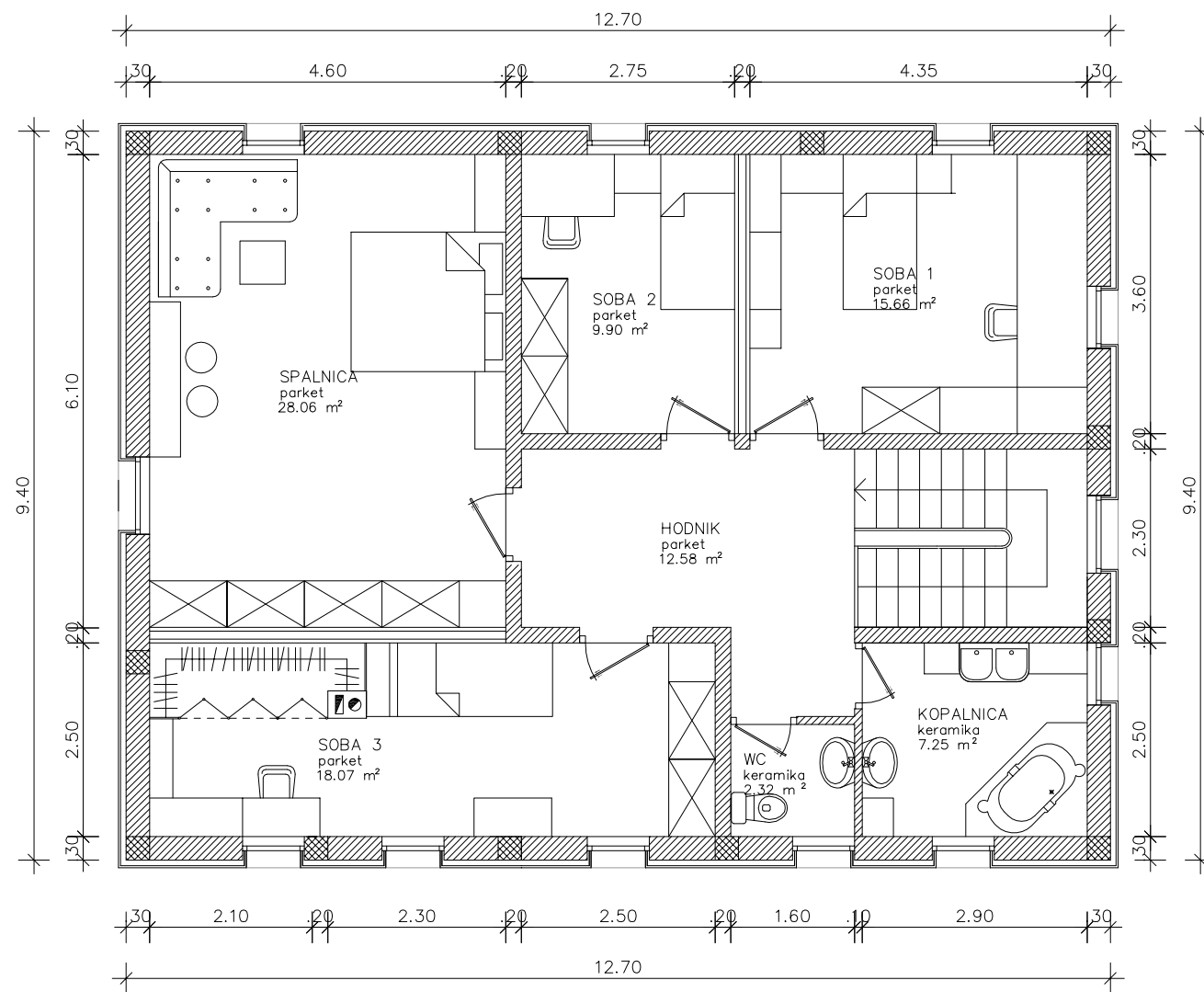
TLORIS MANSARDE
