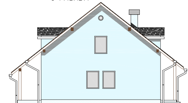
J FASADA
