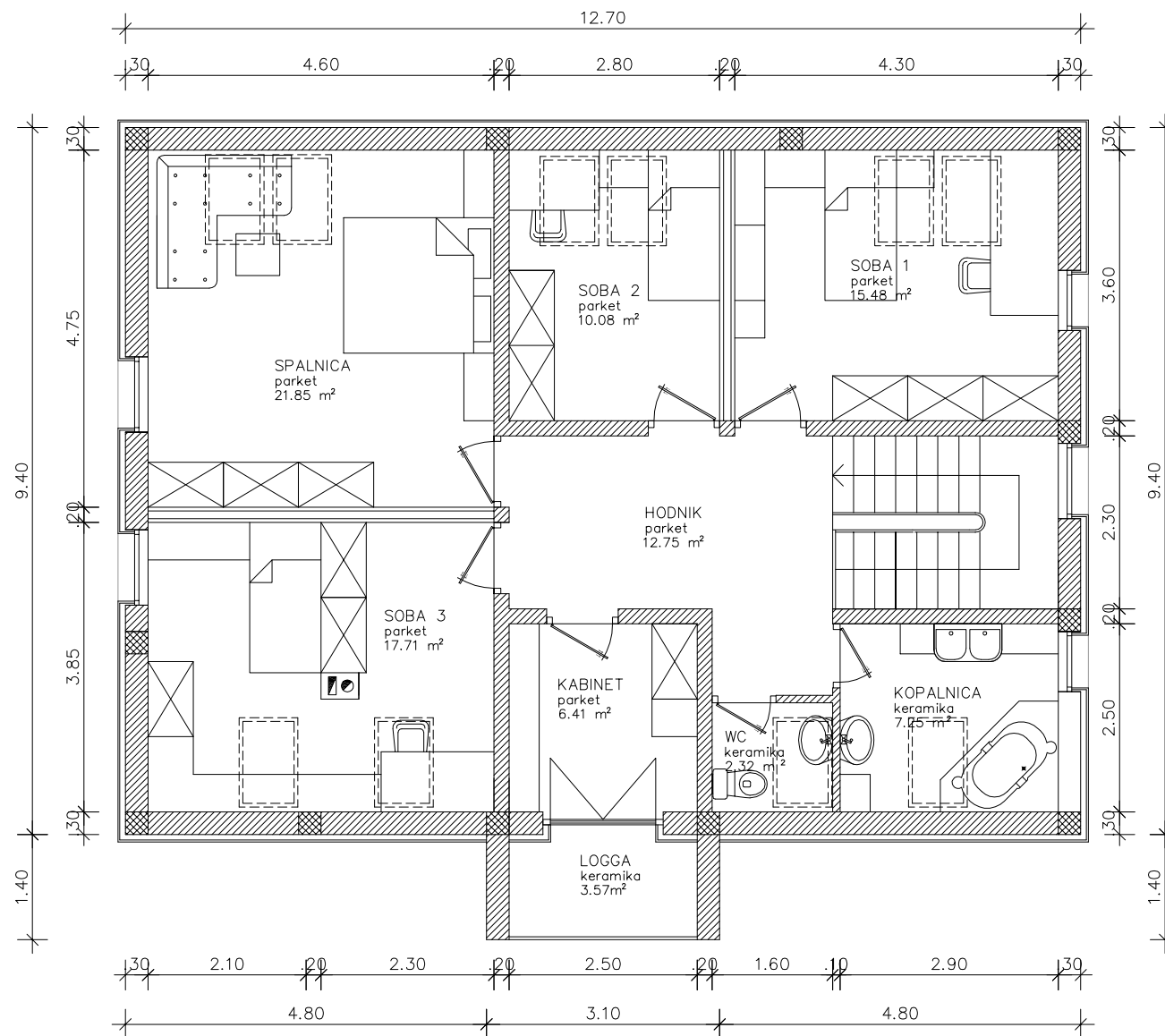
TLORIS MANSARDE
