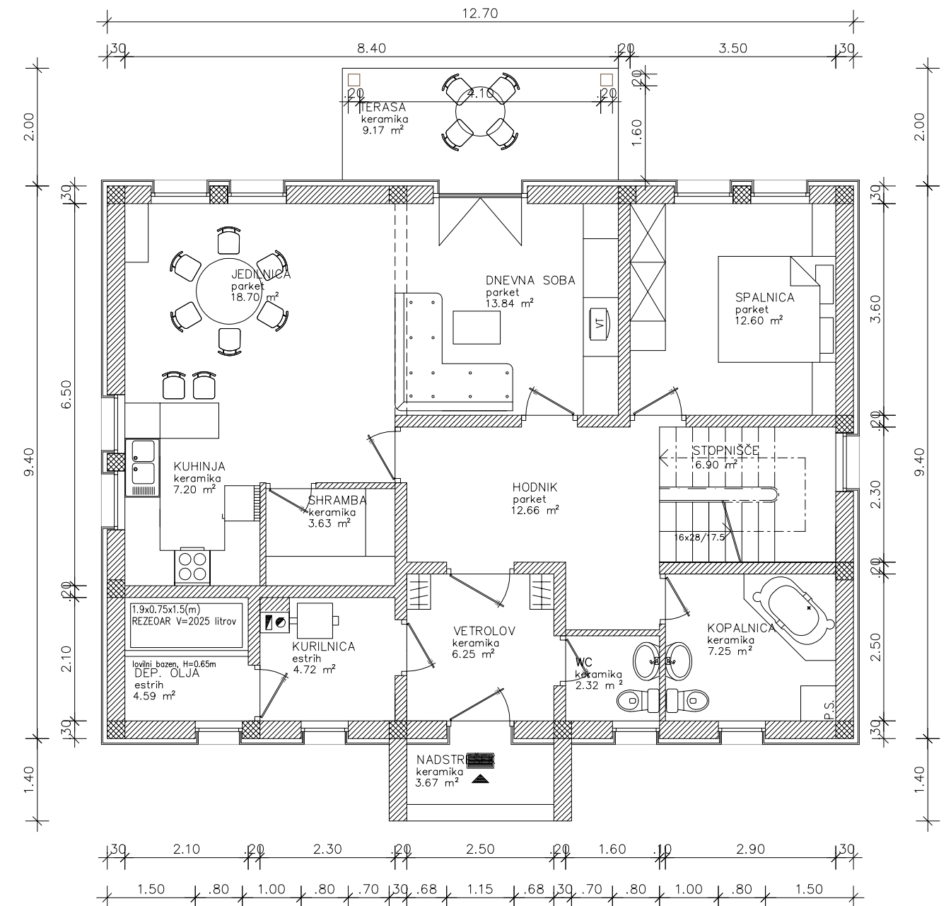
TLORIS PRITLIČJA
