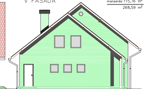
V FASADA
