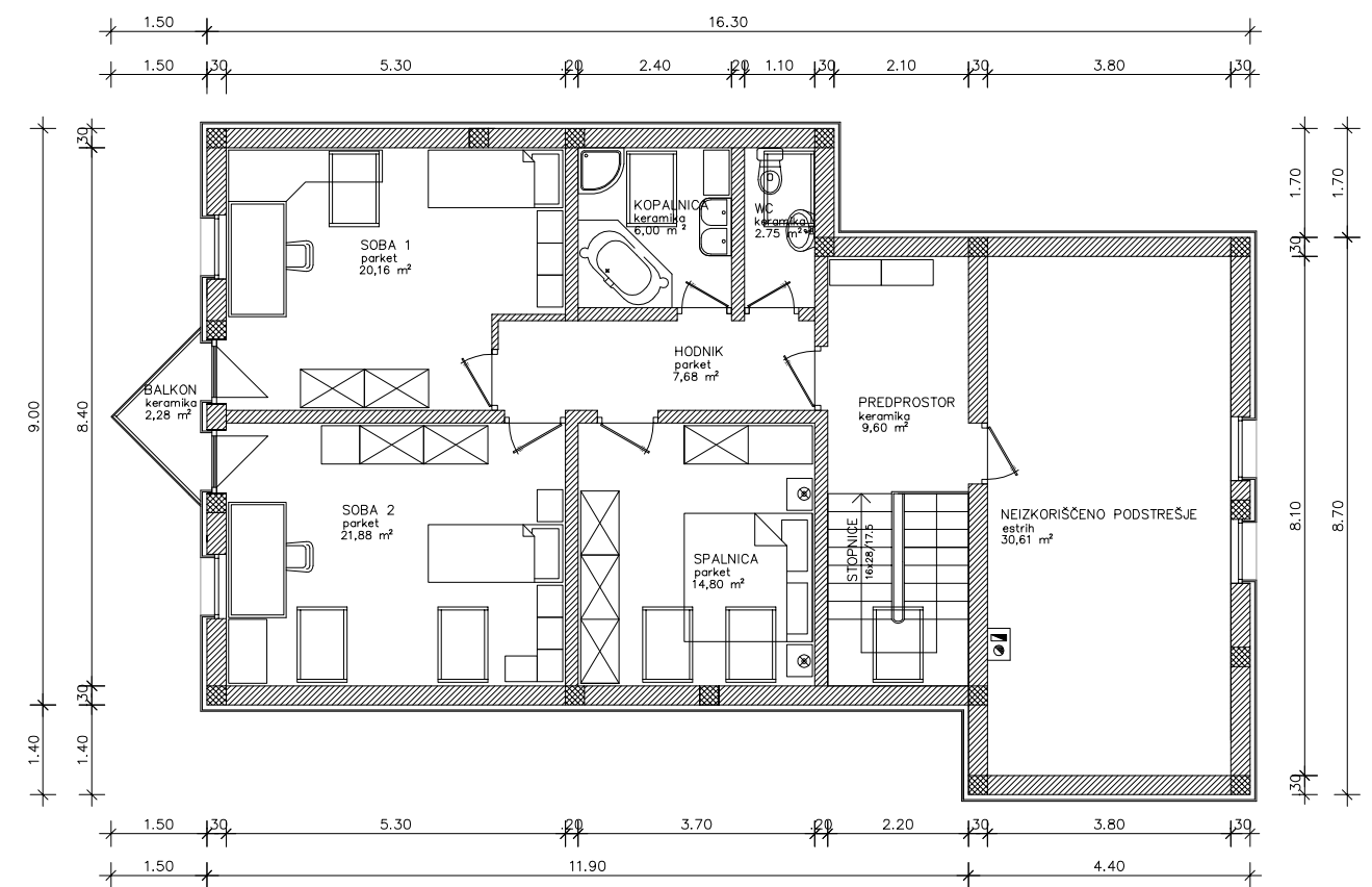
TLORIS MANSARDE
