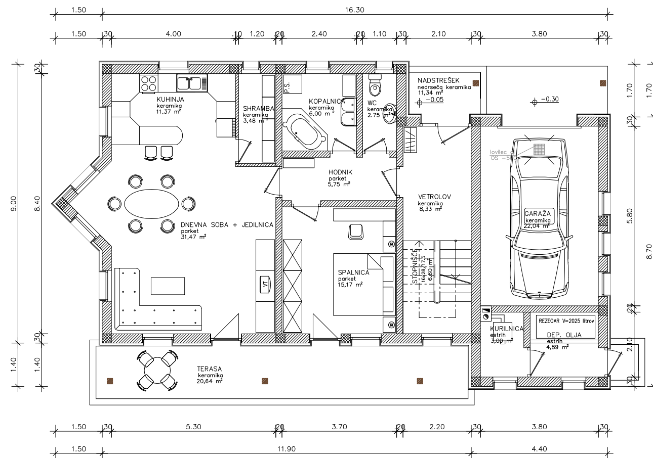
TLORIS PRITLIČJA
