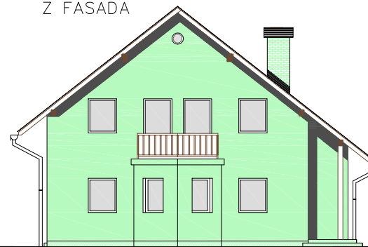
Z FASADA
