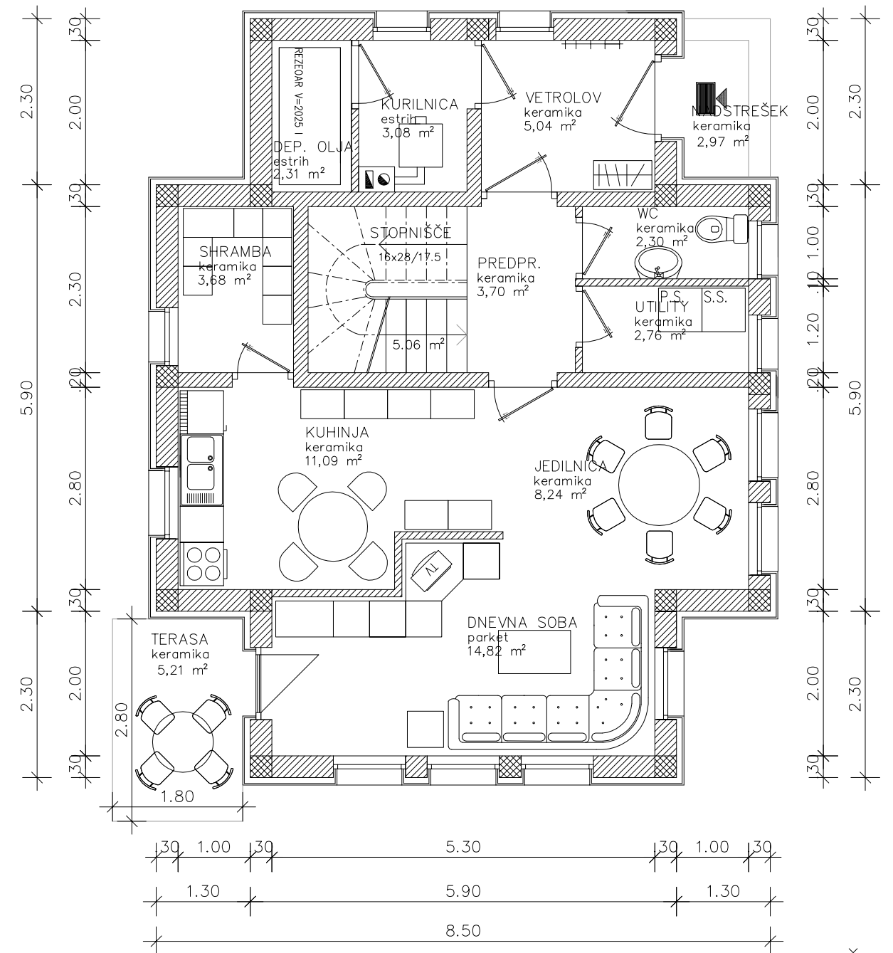
TLORIS PRITLIČJA
