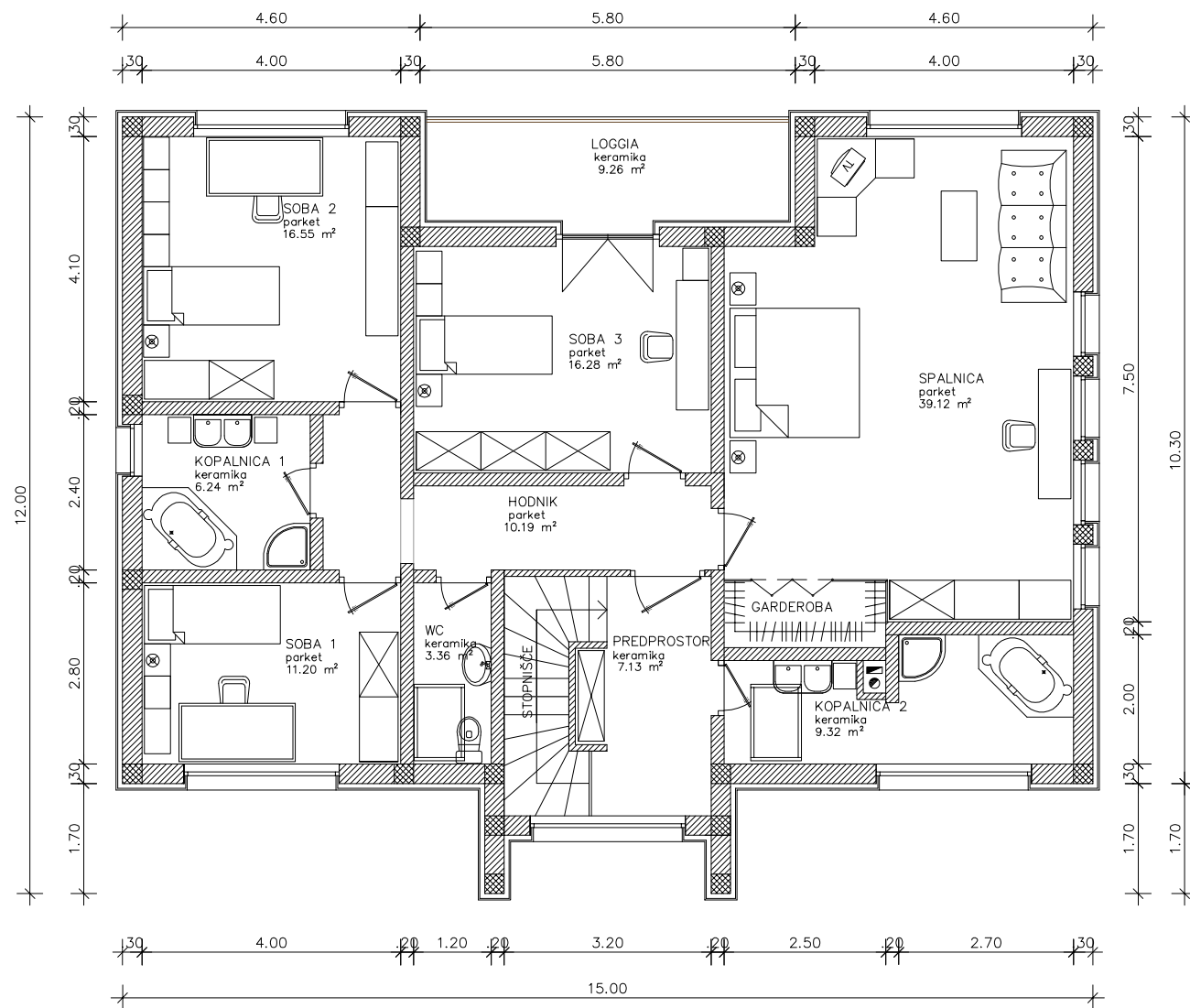
TLORIS MANSARDE
