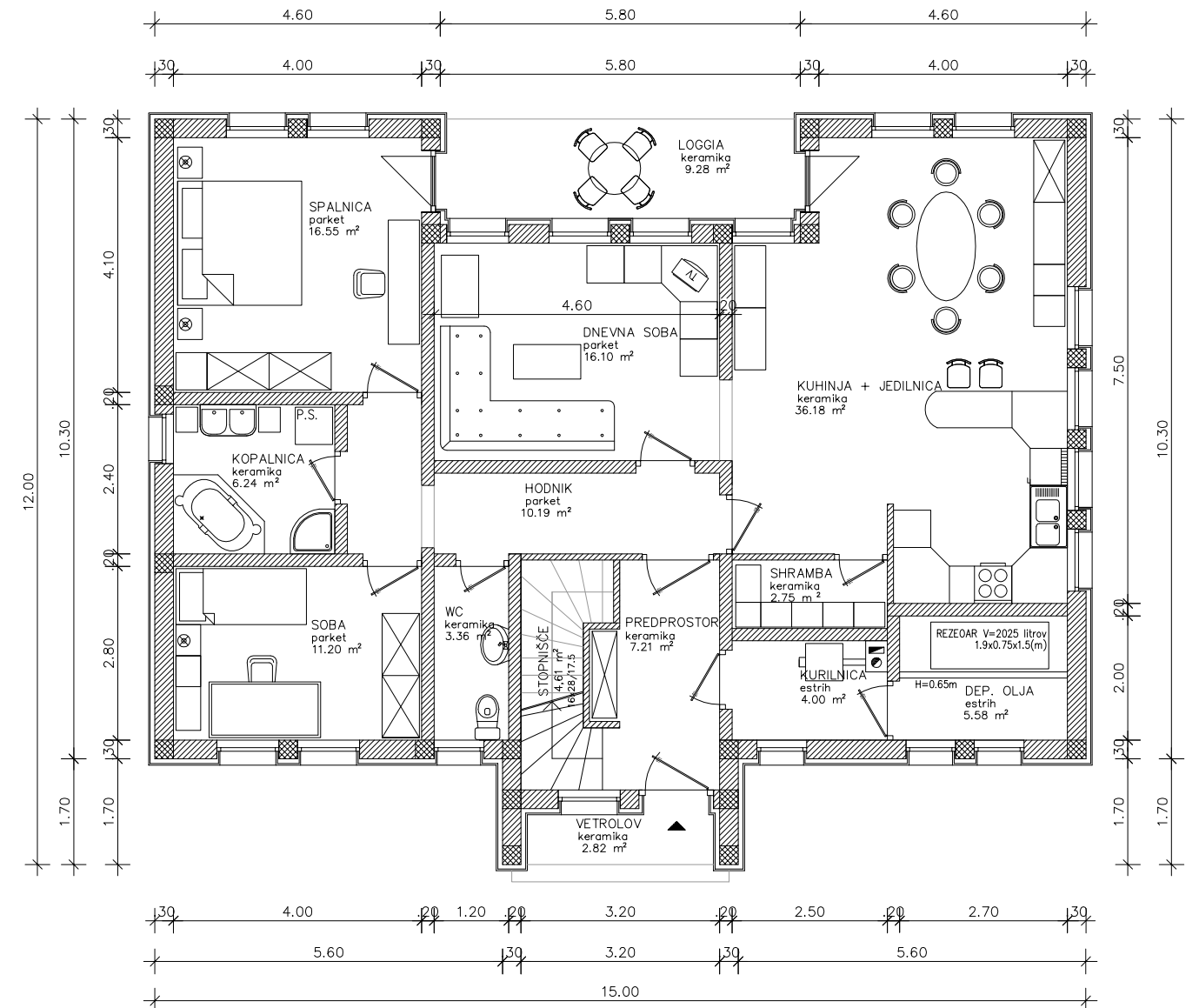
TLORIS PRITLIČJA
