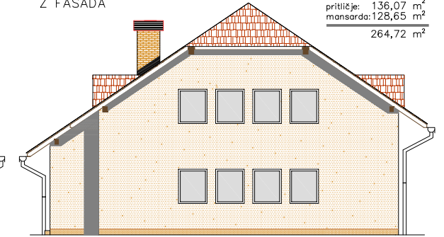
Z FASADA
