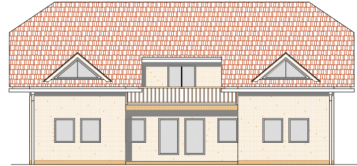
J FASADA
