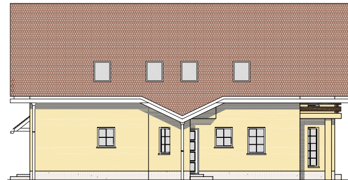
S FASADA
