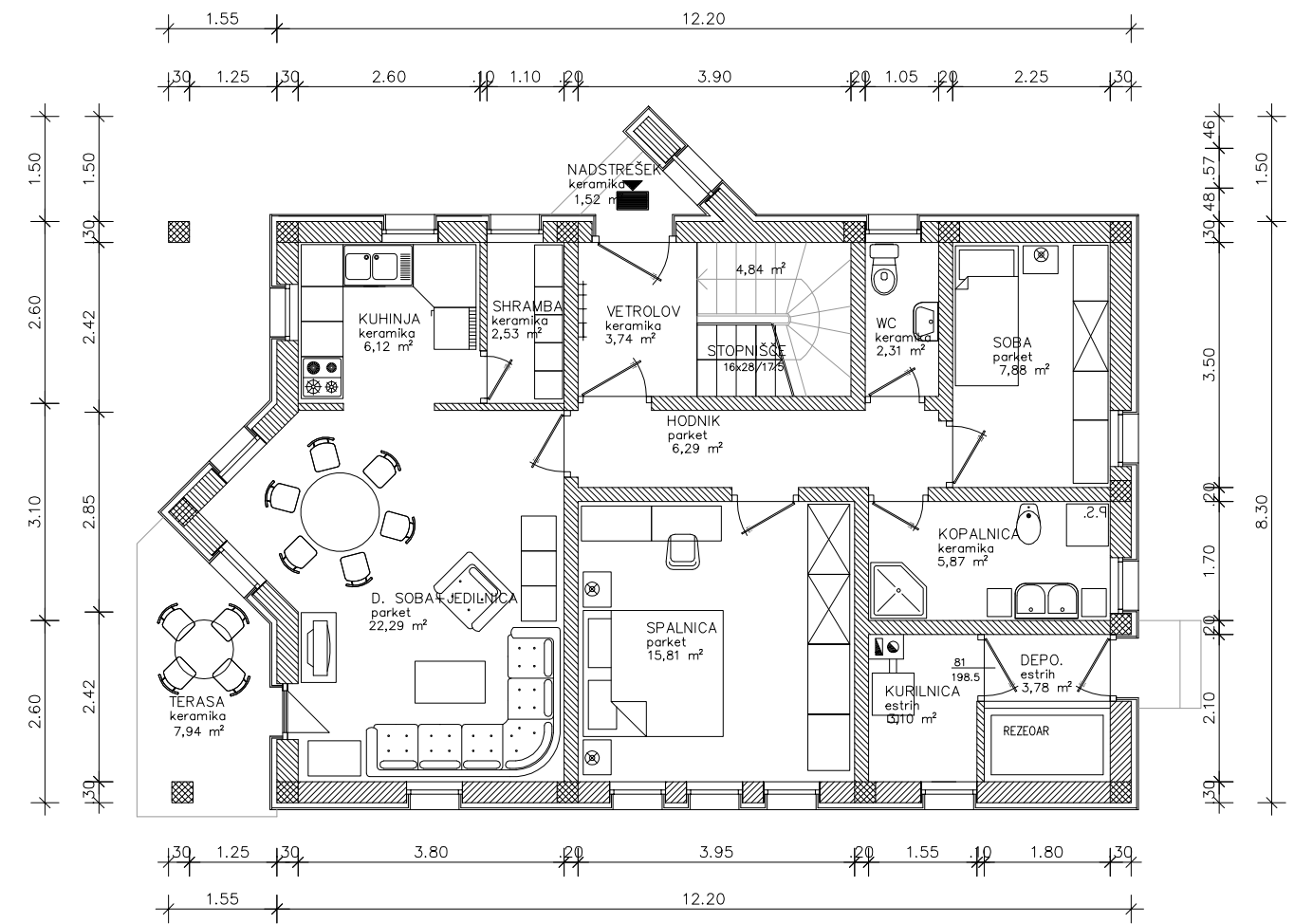
TLORIS PRITLIČJA
