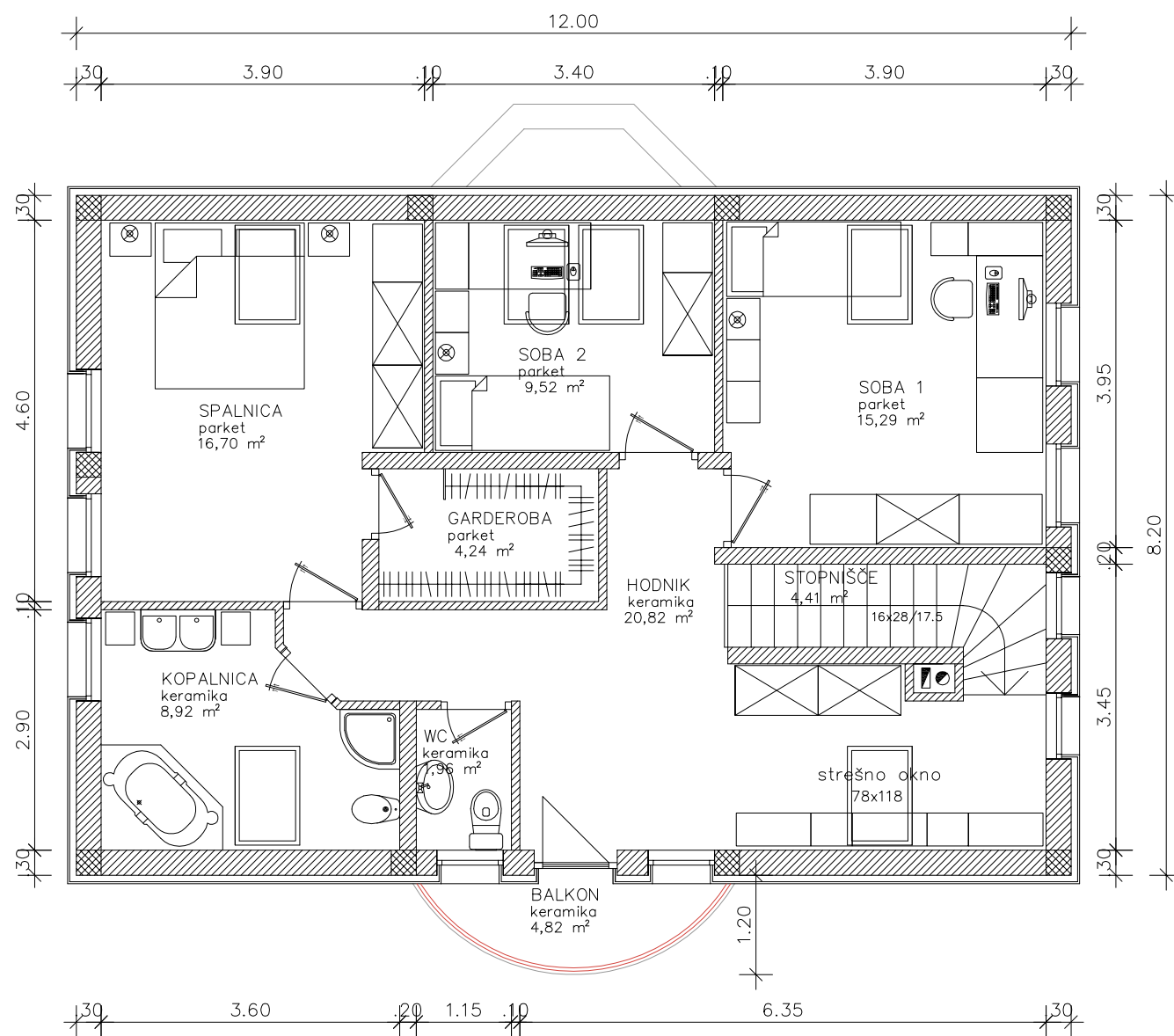
TLORIS MANSARDE
