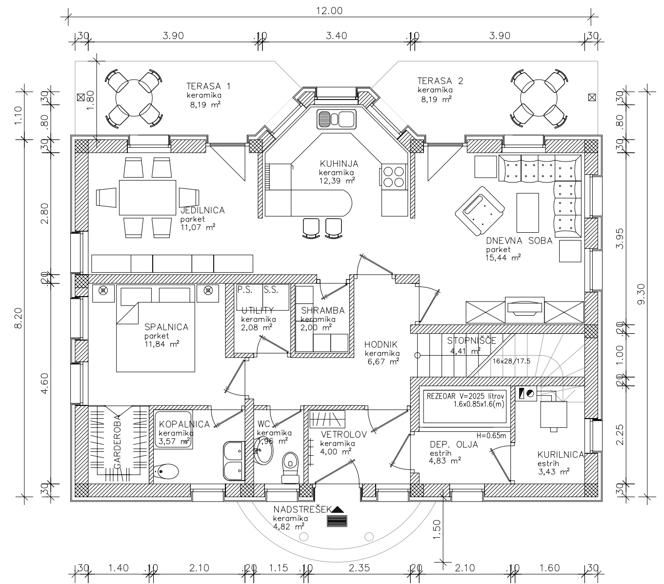
TLORIS PRITLIČJA
