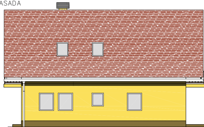
Z FASADA
