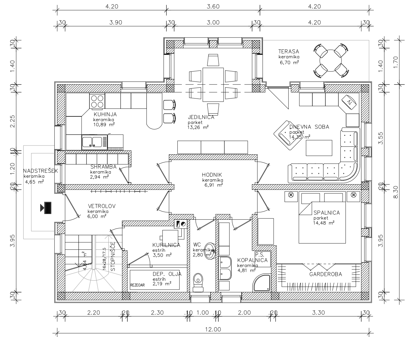
TLORIS PRITLIČJA
