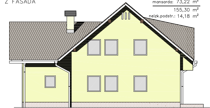
Z FASADA
