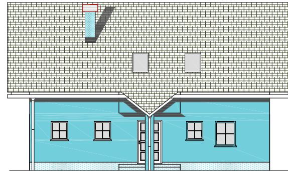
S FASADA
