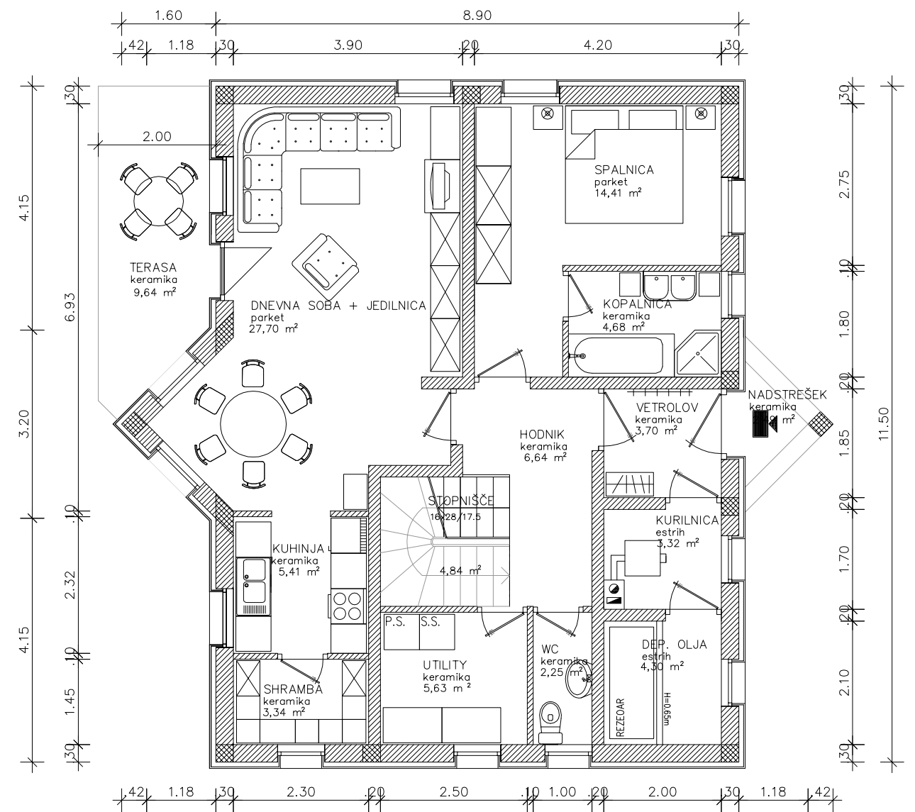
TLORIS PRITLIČJA
