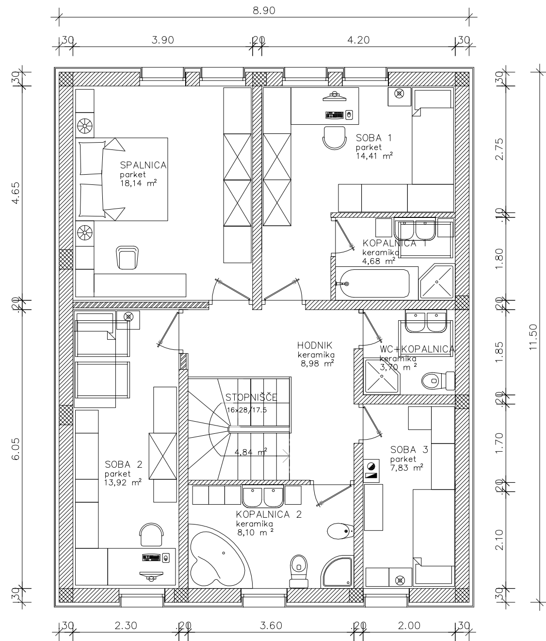
TLORIS MANSARDE
