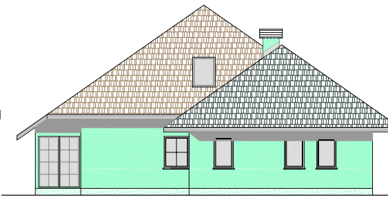
severovzhodna fasada
