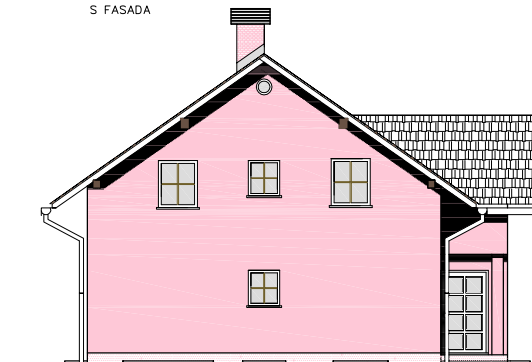
S FASADA
