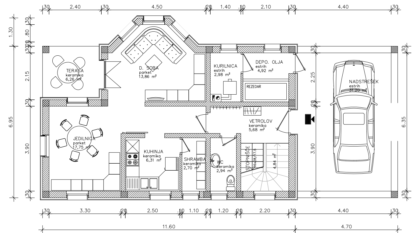
TLORIS PRITLIČJA
