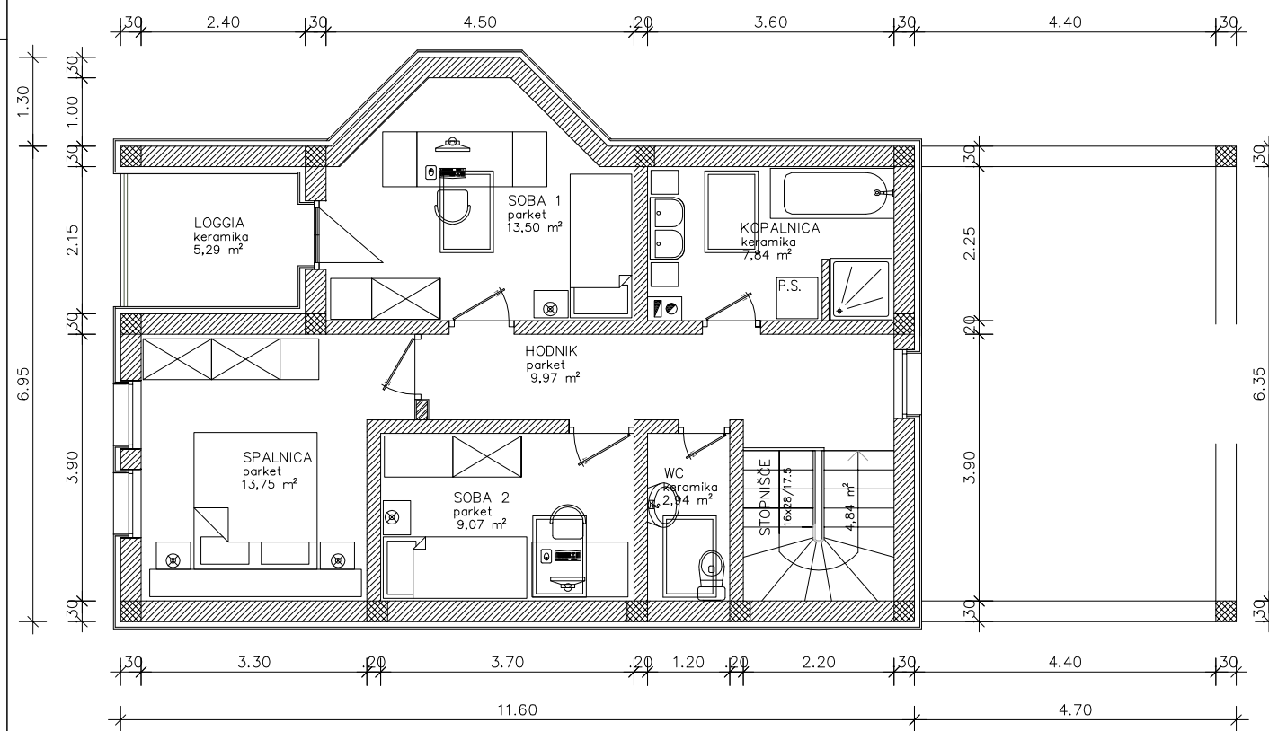
TLORIS MANSARDE
