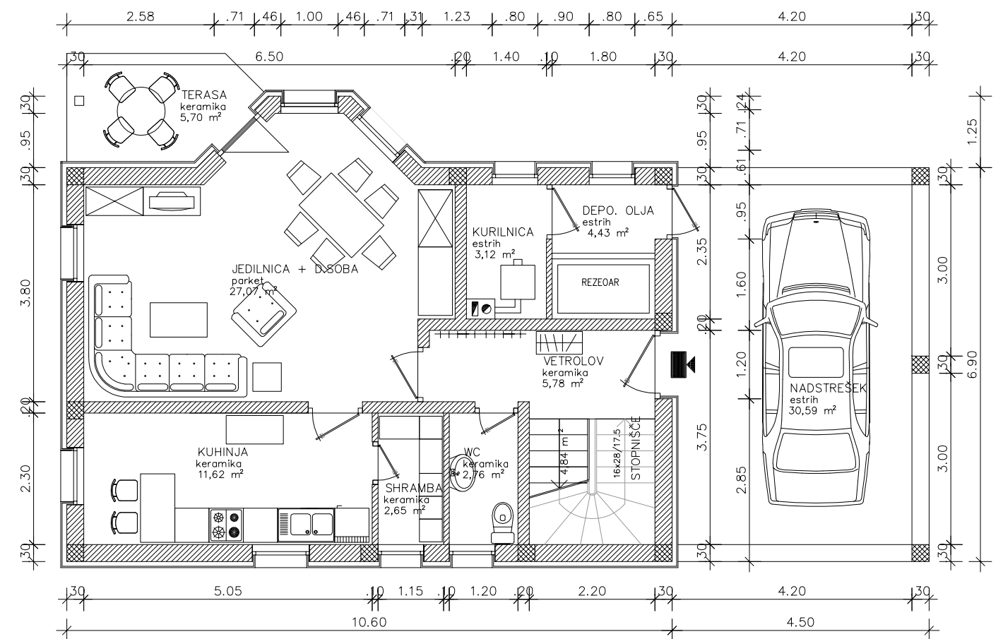
TLORIS PRITLIČJA
