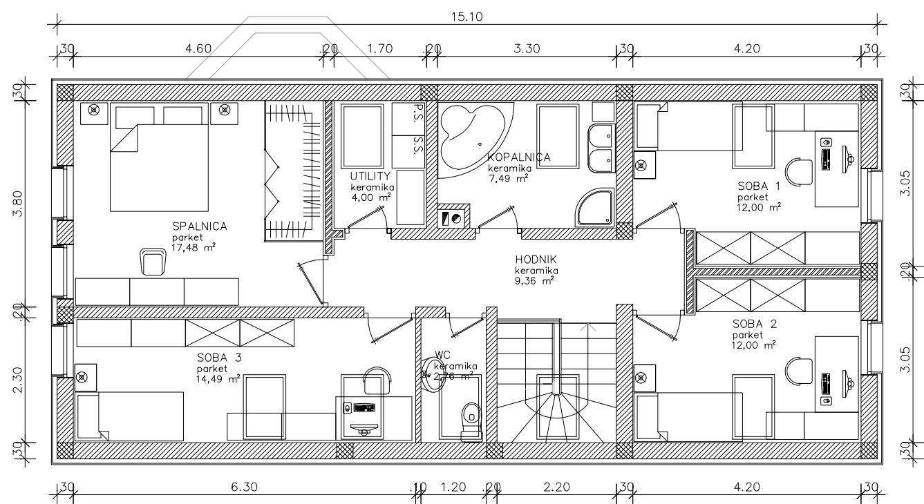
TLORIS MANSARDE
