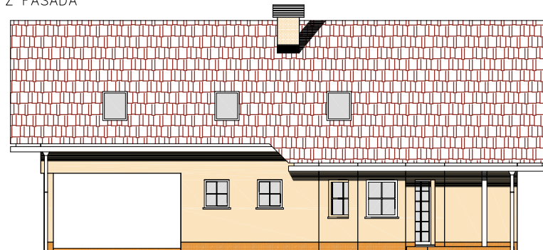
Z FASADA
