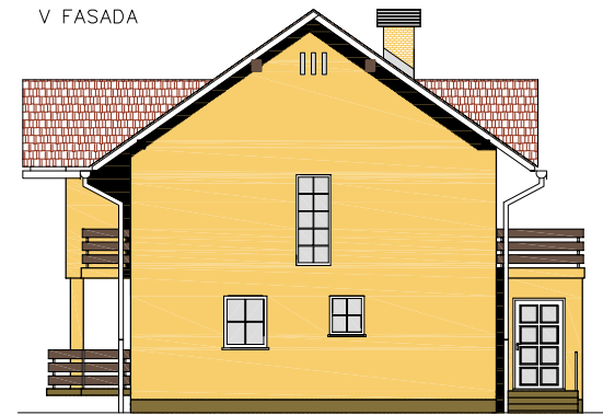
V FASADA
