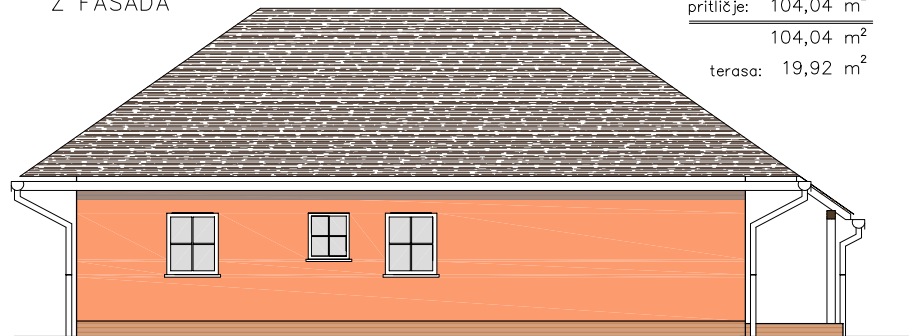
Z FASADA
