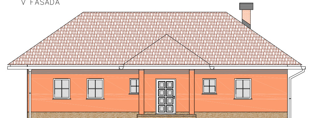
V FASADA
