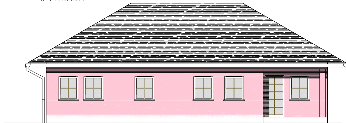
J FASADA
