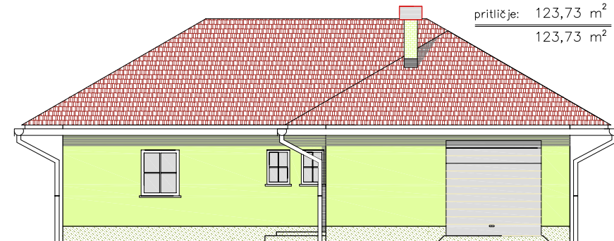
S FASADA
