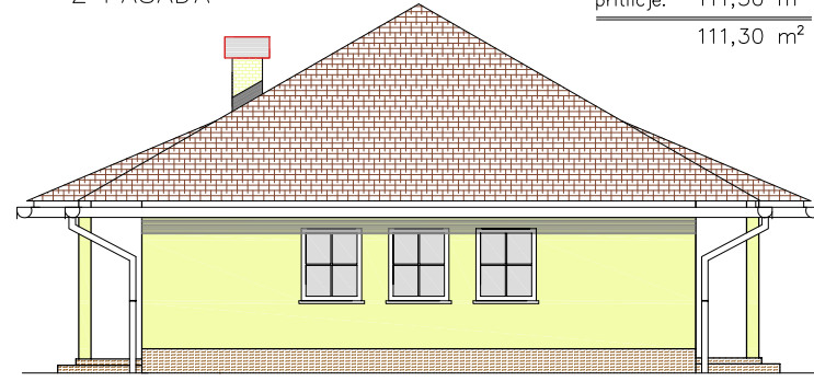
Z FASADA
