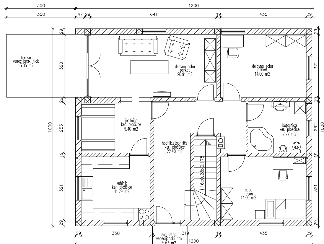
PRITIČJE
