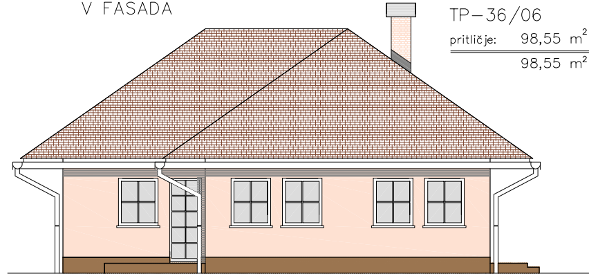
V FASADA
