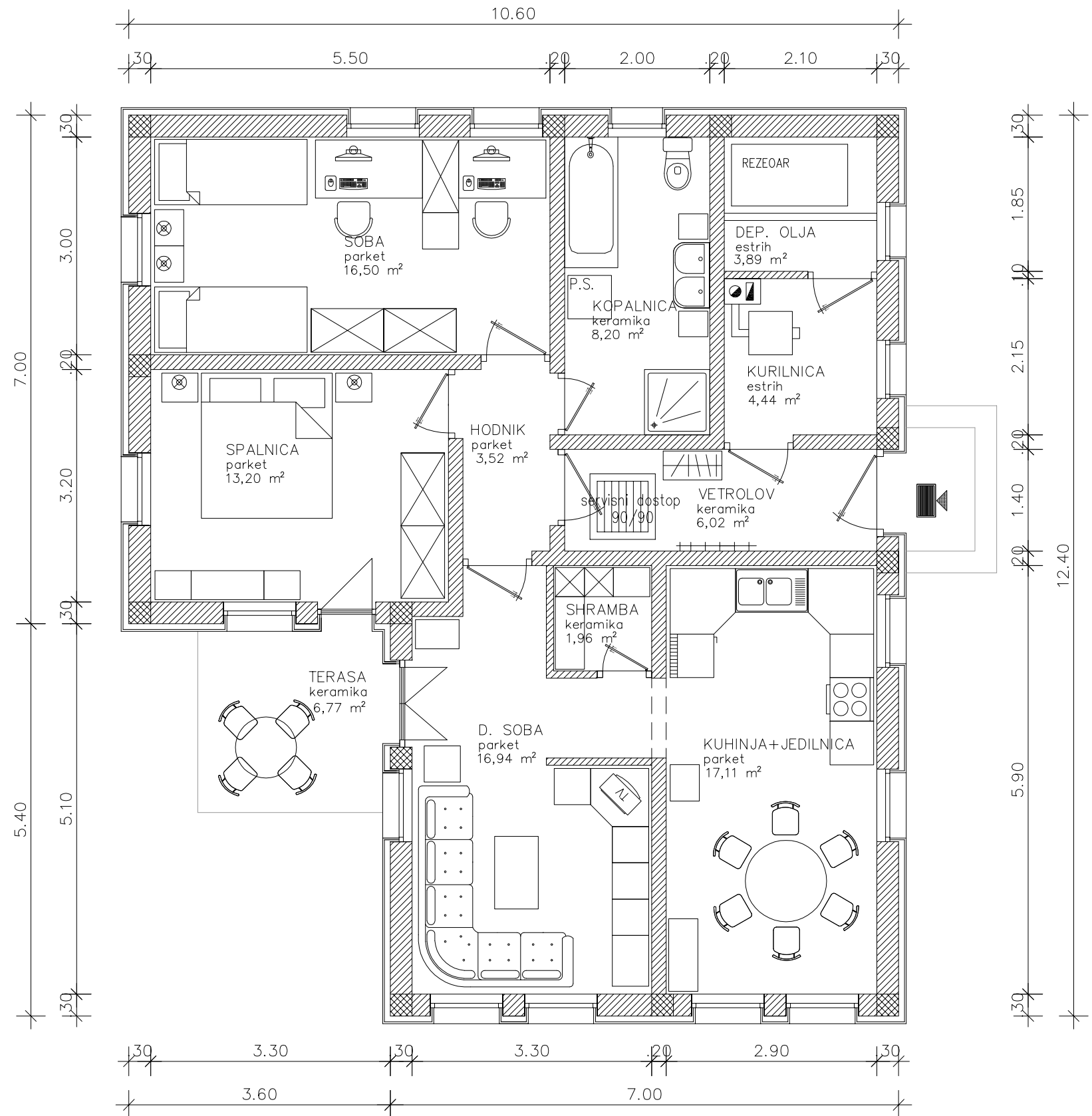
TLORIS PRITLIČJA
