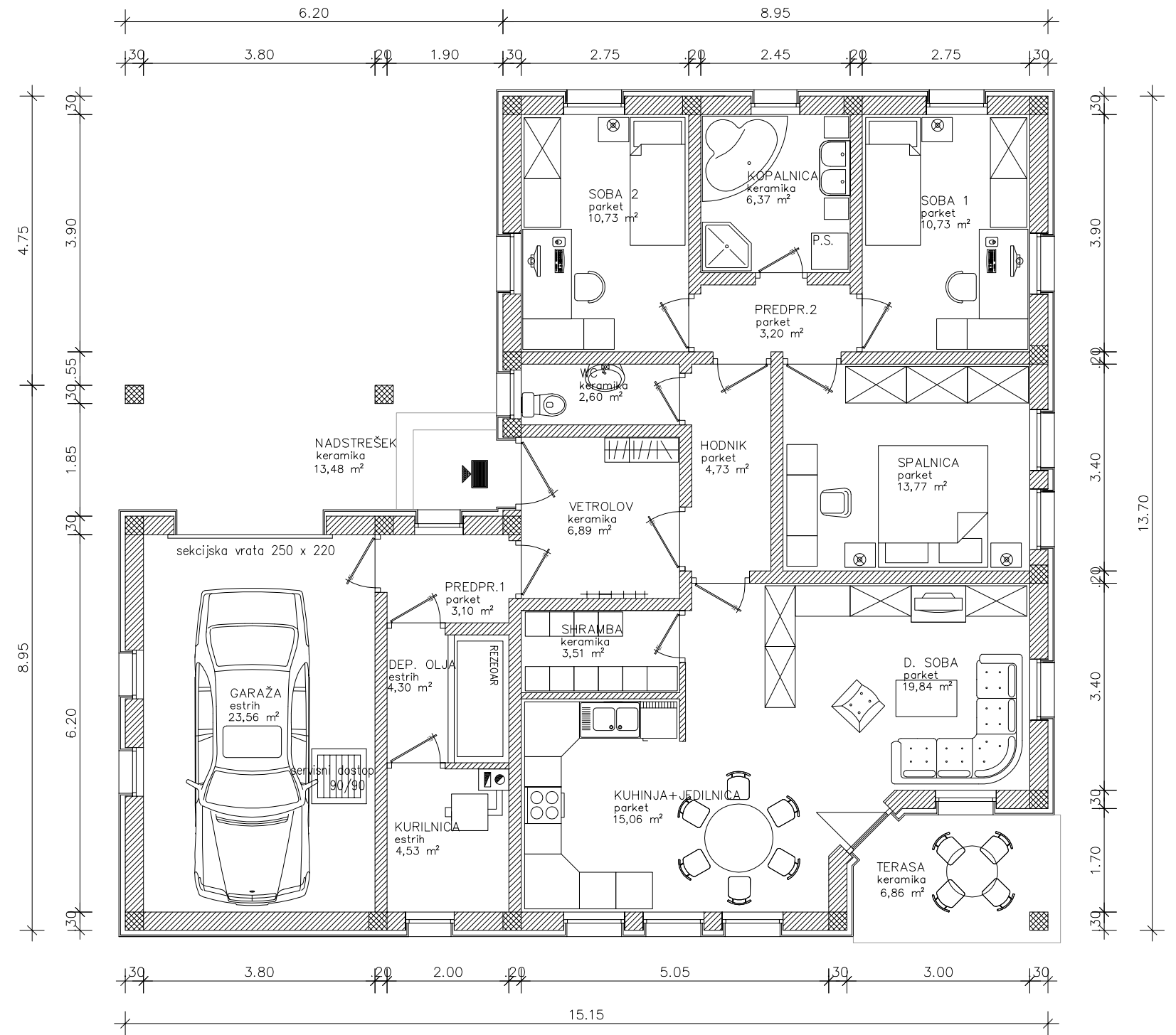
TLORIS PRITLIČJA
