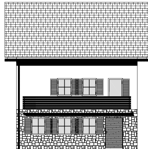
J FASADA
