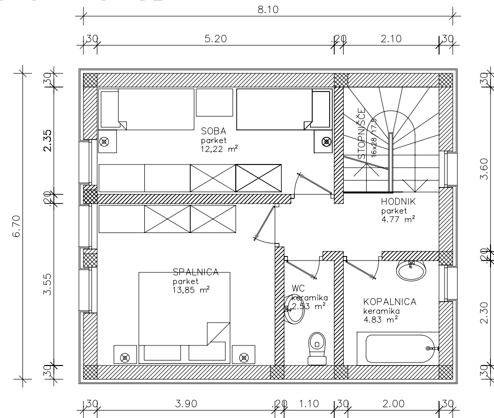
TLORIS MANSARDE
