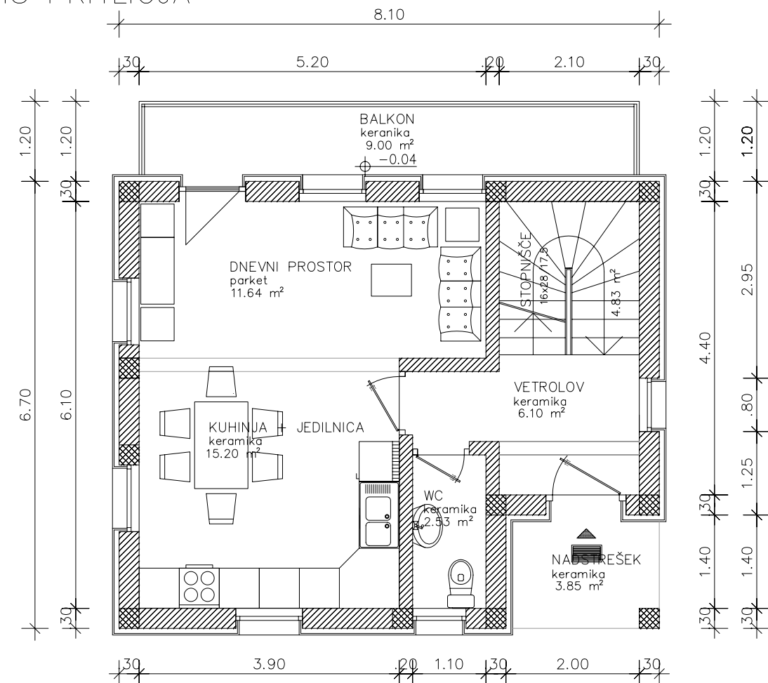
TLORIS PRITLIČJA
