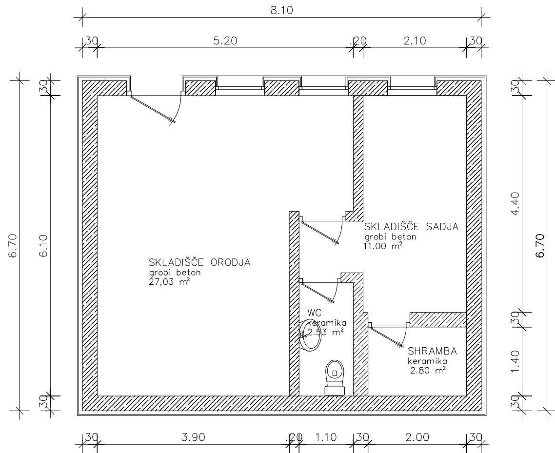
TLORIS KLETI
