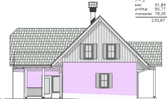
VZHODNA FASADA
