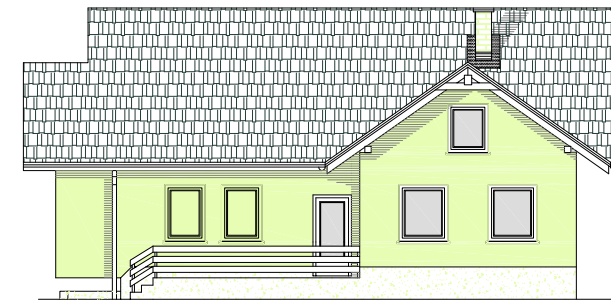
JUŽNA FASADA
