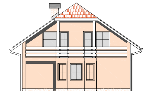
ZAHODNA FASADA
