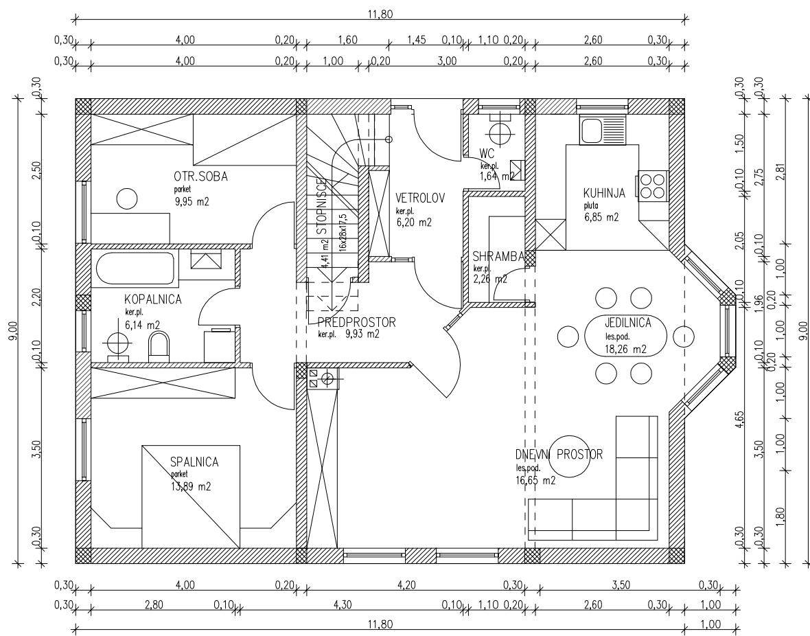
TLORIS PRITLIČJA
