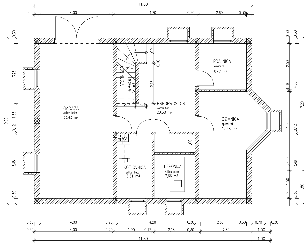
TLORIS KLETI
