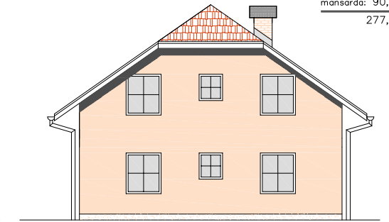
VZHODNA FASADA
