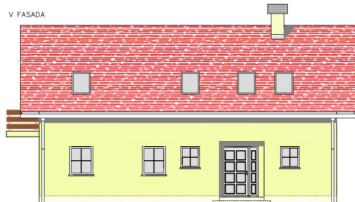
J FASADA
