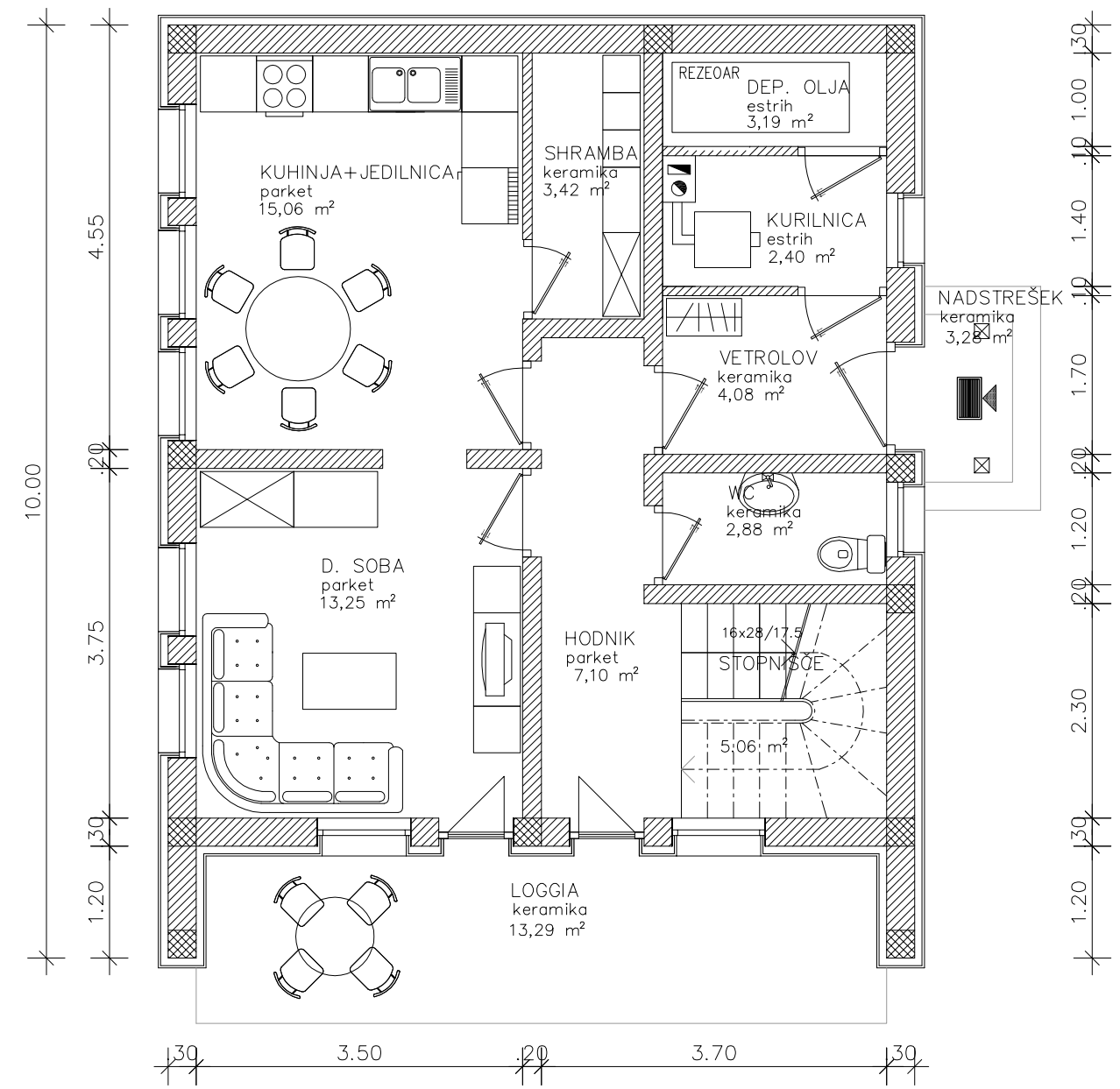
TLORIS PRITLIČJA
