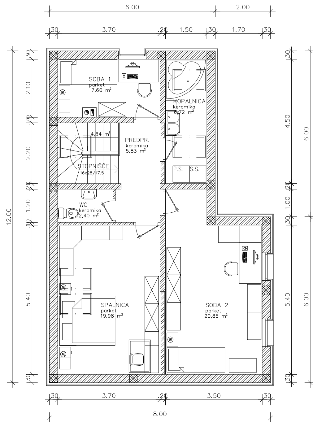
TLORIS MANSARDE
