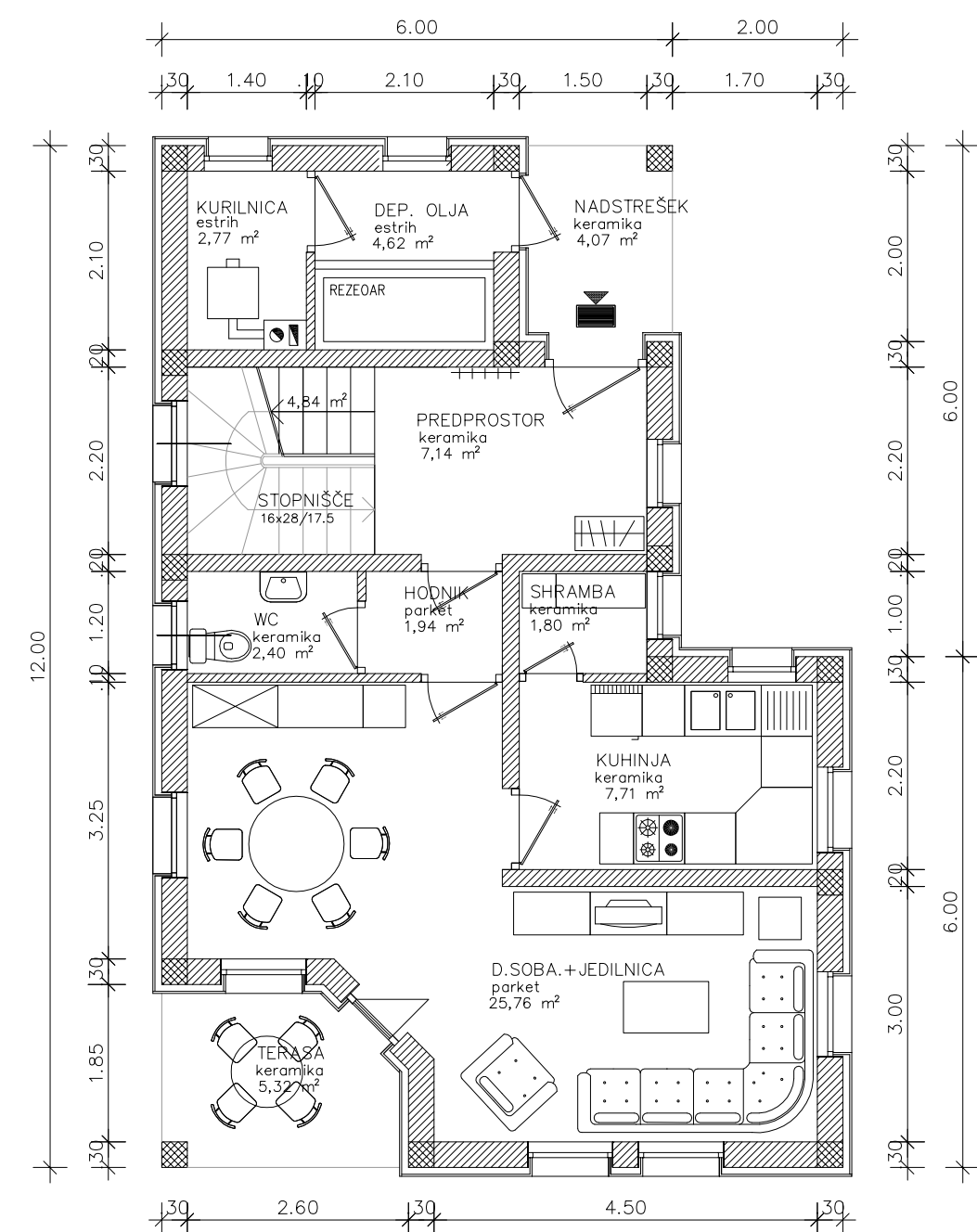
TLORIS PRITLIČJA
