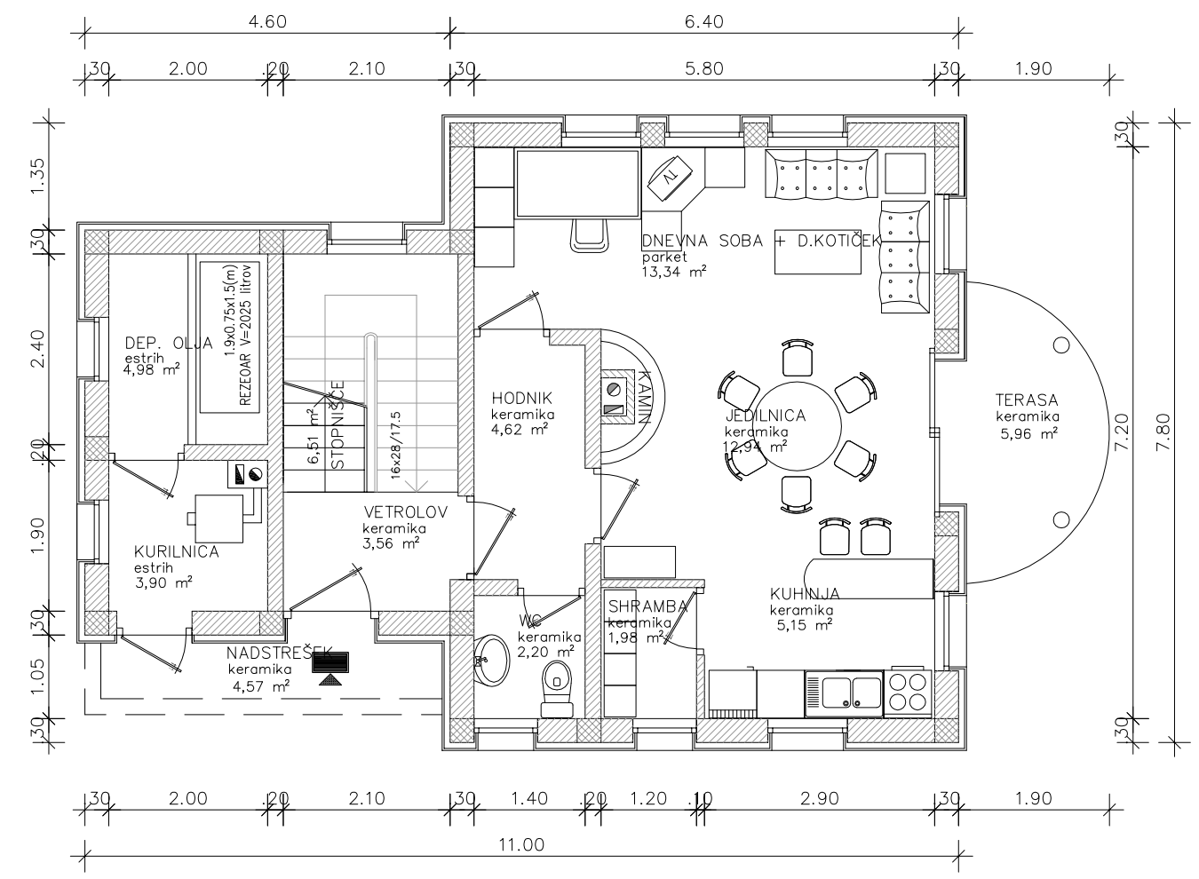
TLORIS PRITLIČJA
