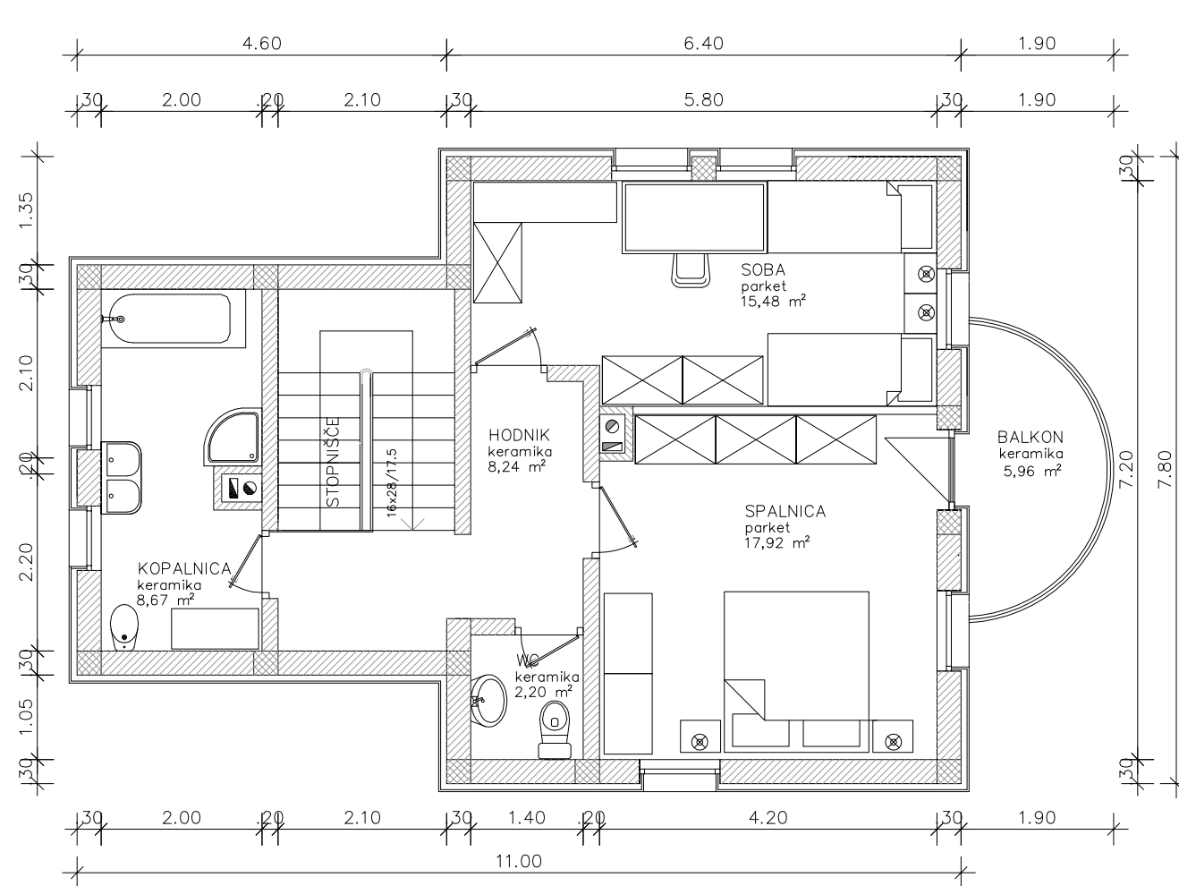
TLORIS MANSARDE
