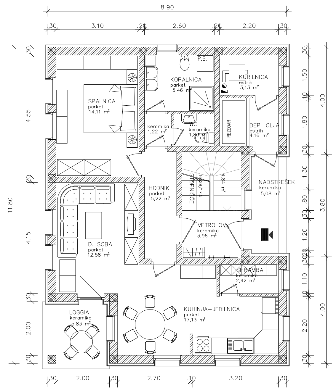
TLORIS PRITLIČJA
