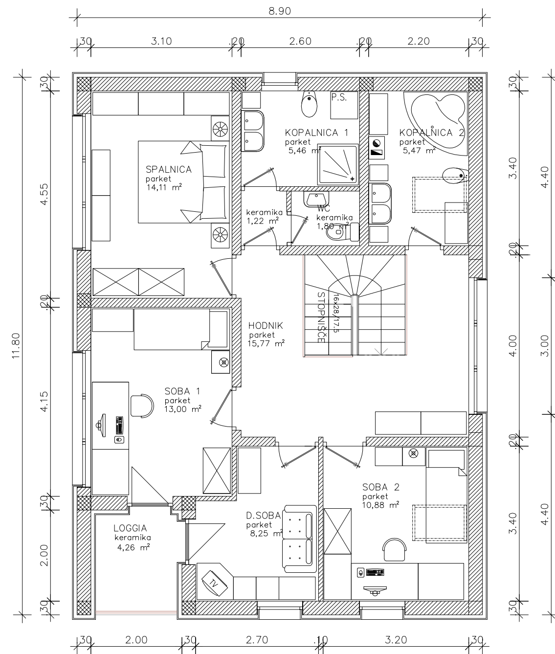
TLORIS MANSARDE
