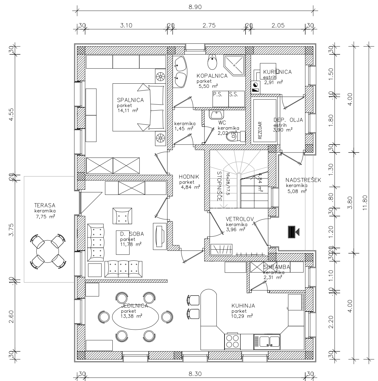
TLORIS PRITLIČJA
