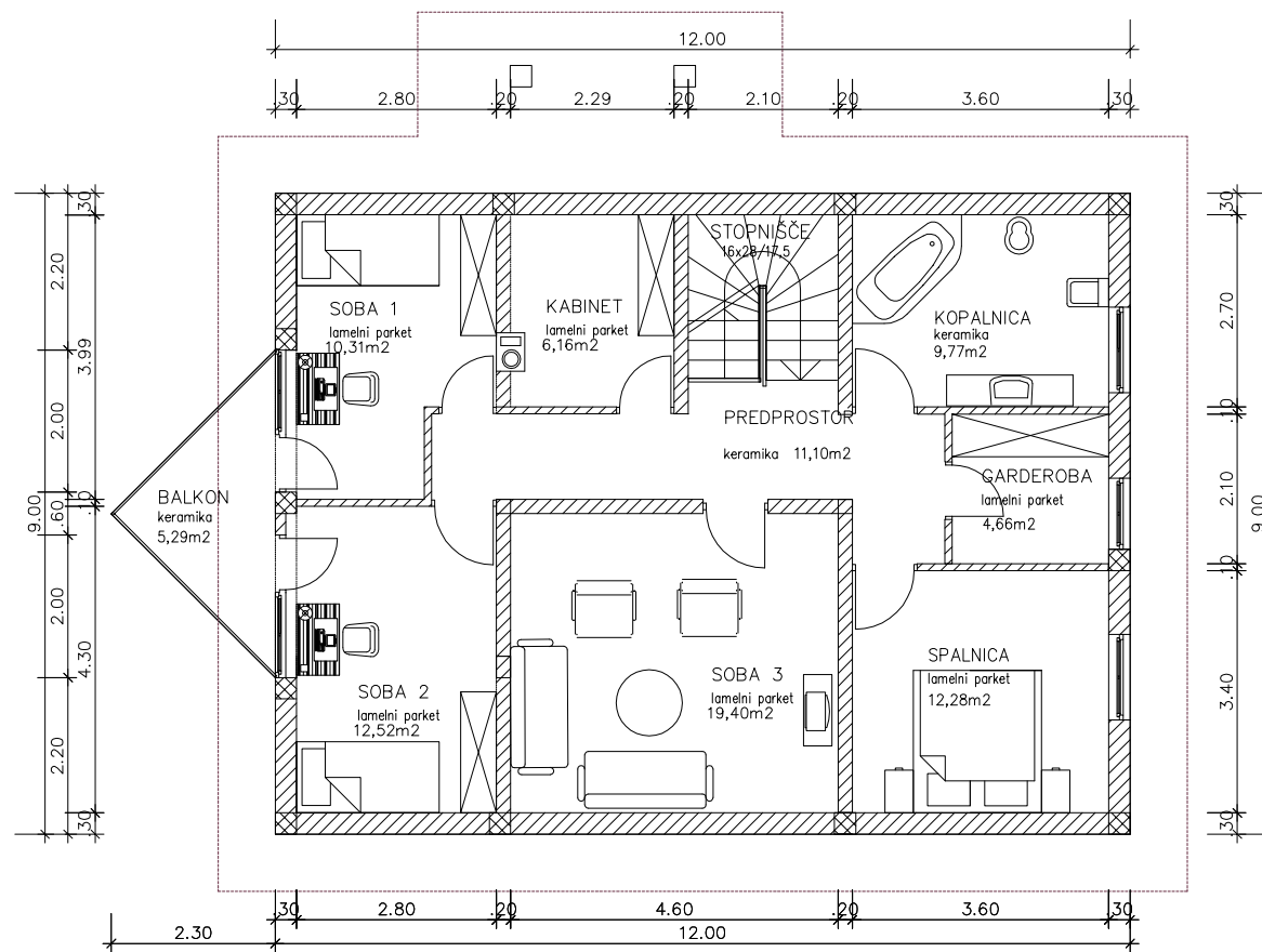
TLORIS MANSARDE
