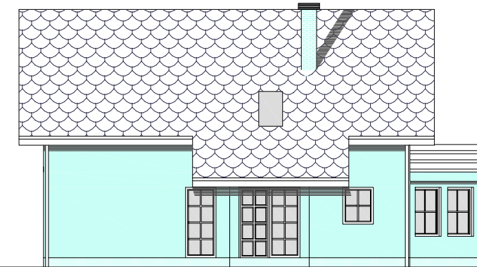
ZAHODNA FASADA
