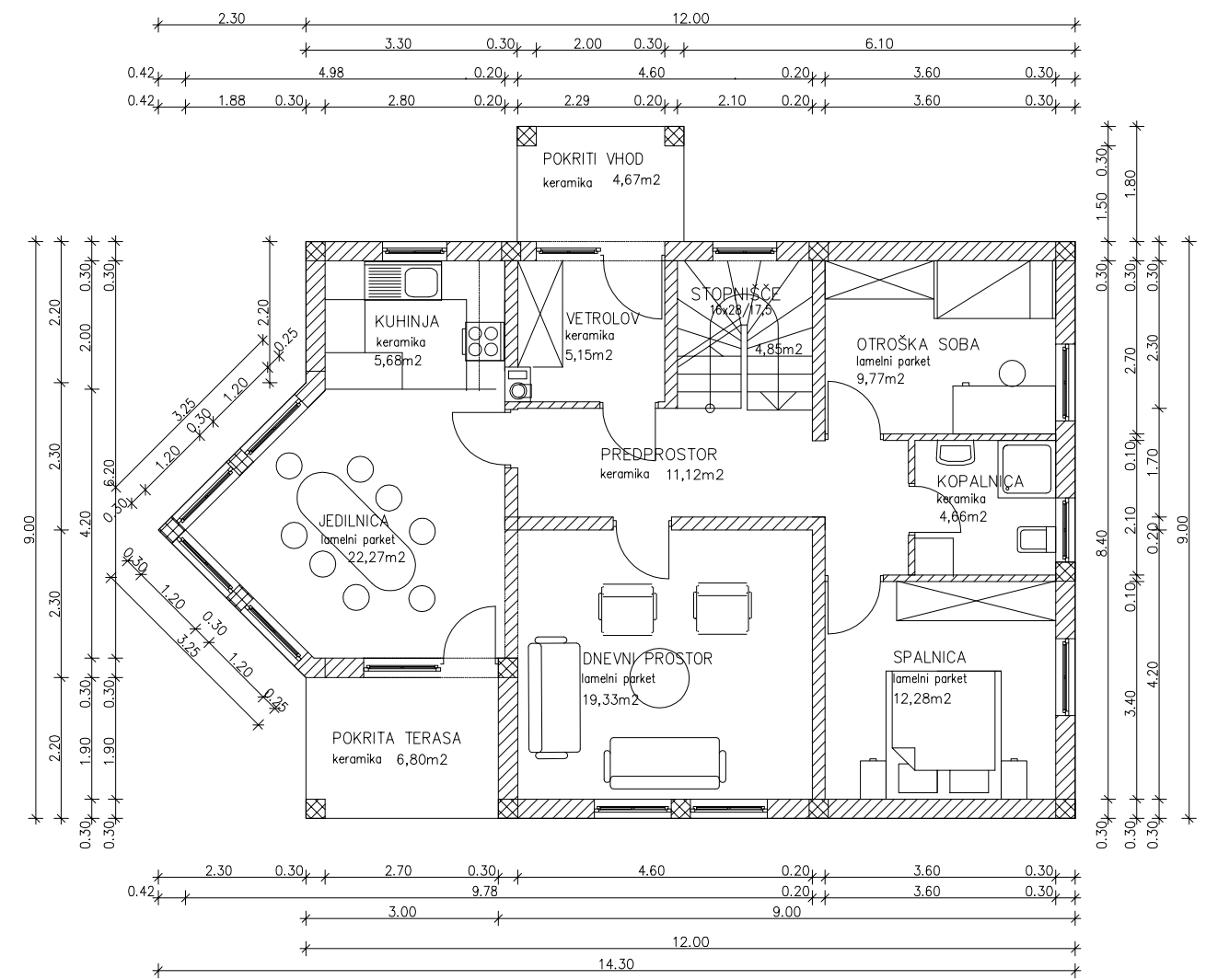
TLORIS PRITLIČJA
