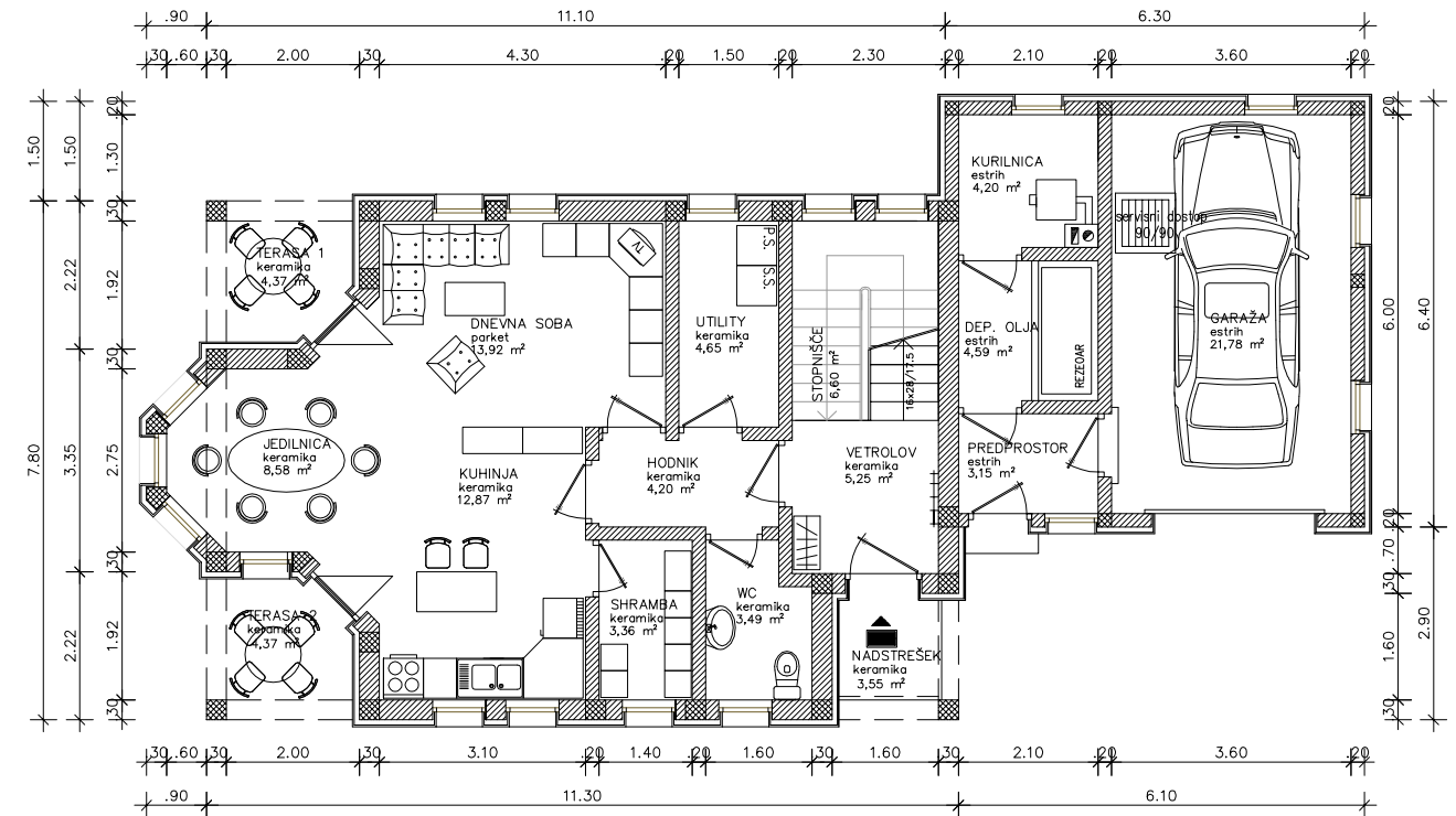
TLORIS PRITLIČJA
