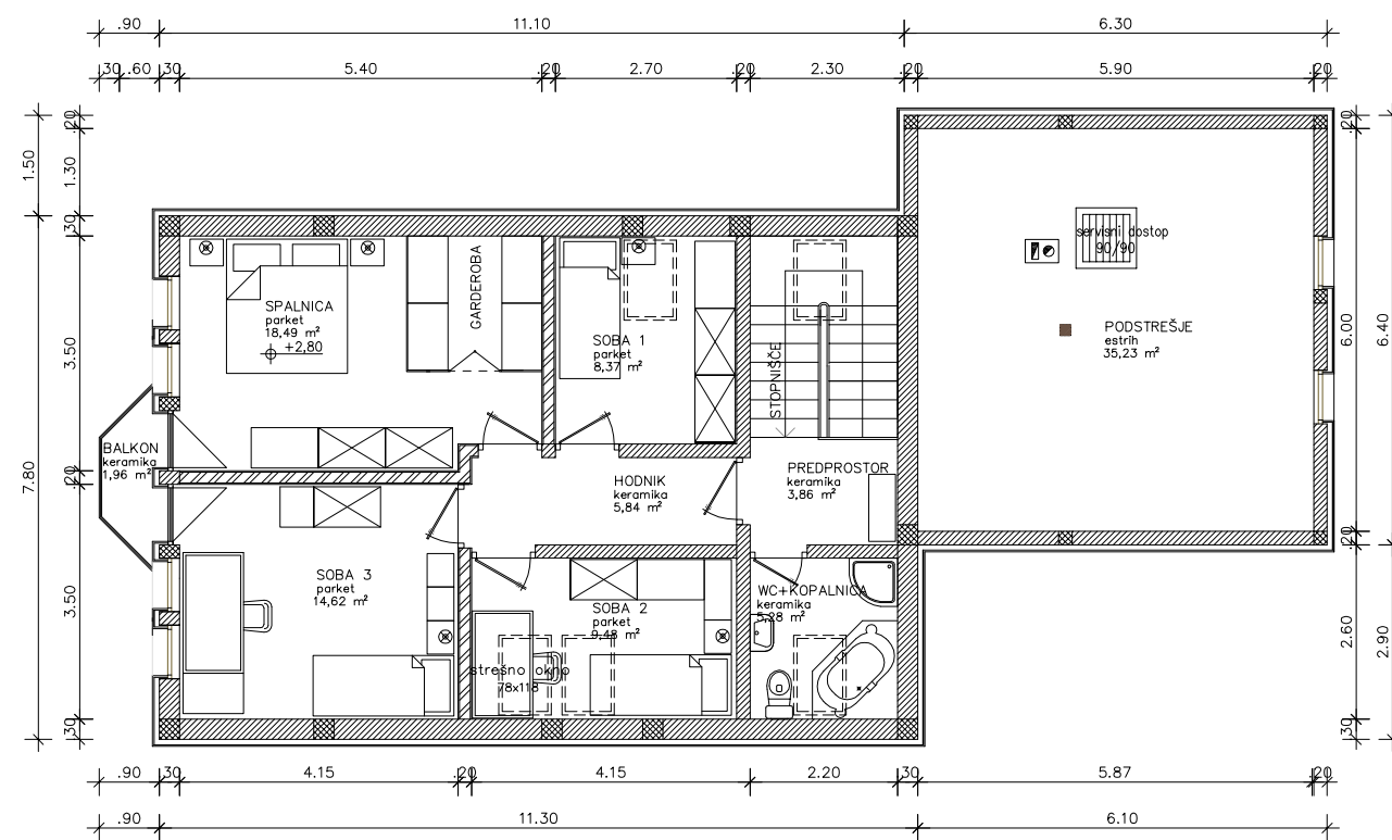
TLORIS MANSARDE
