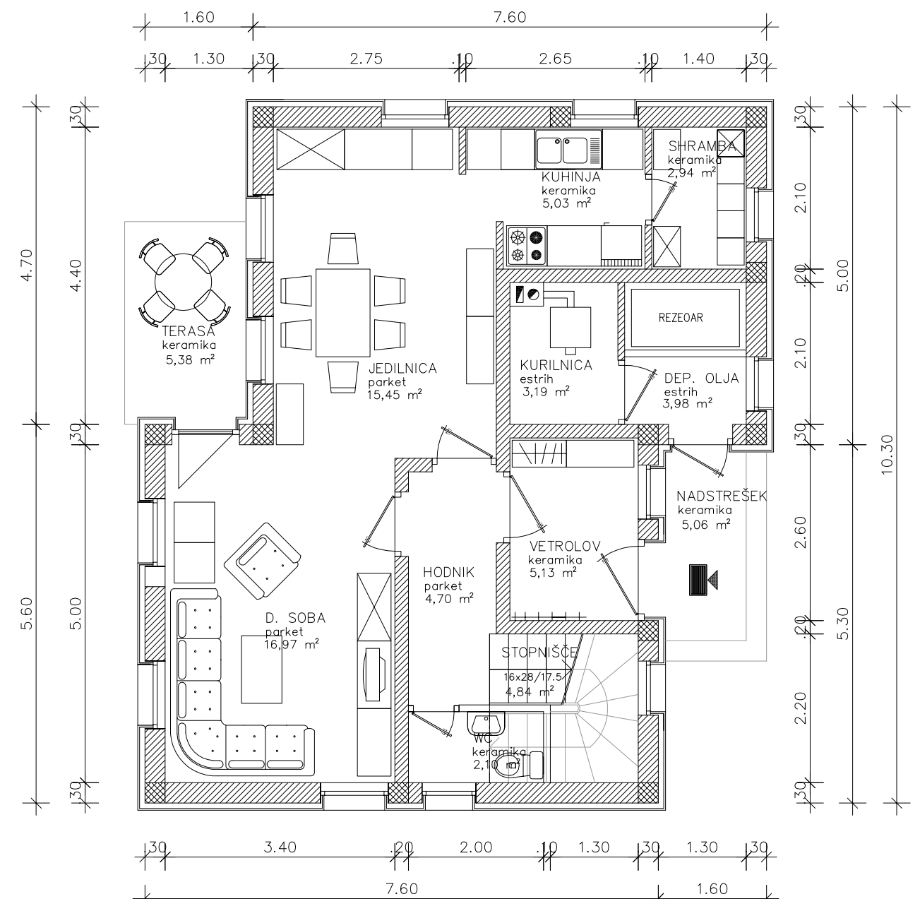
TLORIS PRITLIČJA
