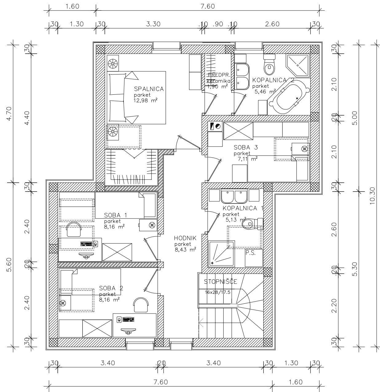
TLORIS MANSARDE
