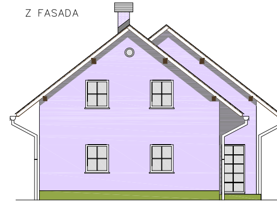
V FASADA
