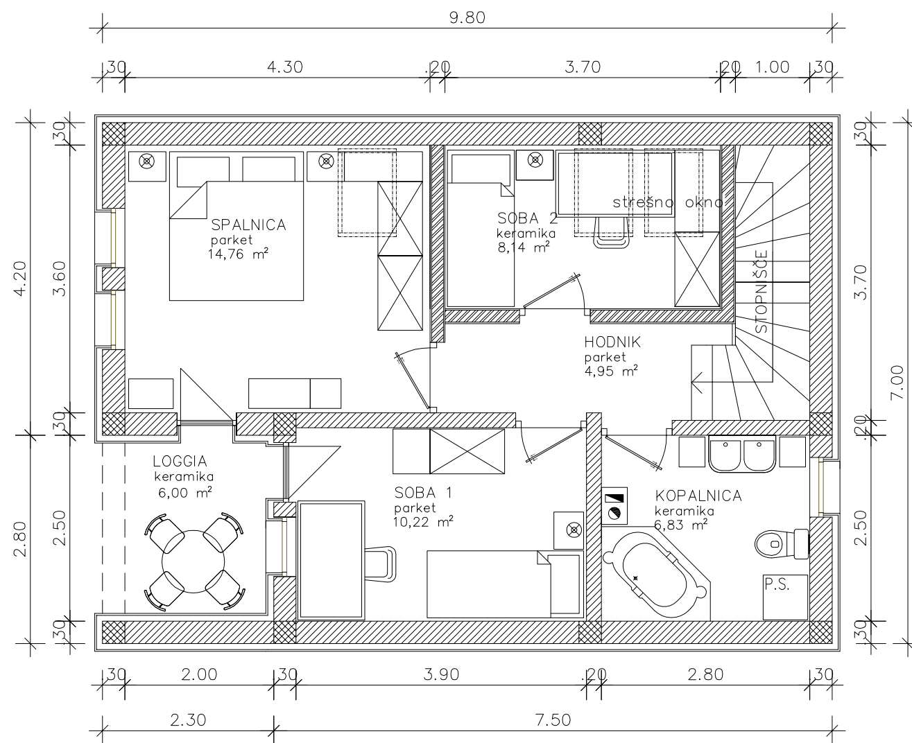
TLORIS MANSARDE
