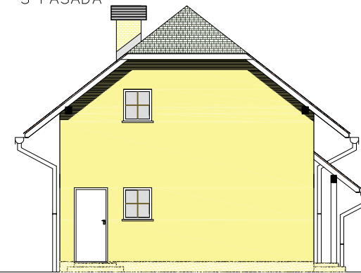
S FASADA
