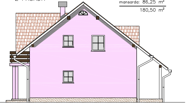
Z FASADA
