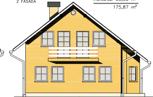
Z FASADA
