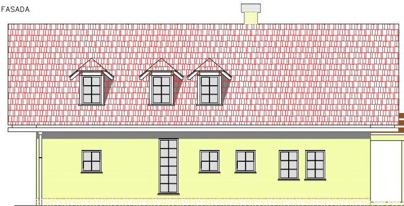
Z FASADA
