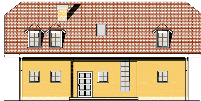
S FASADA
