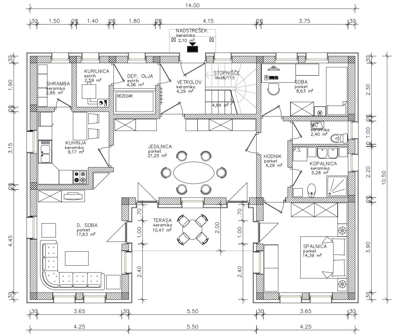
TLORIS PRITLIČJA
