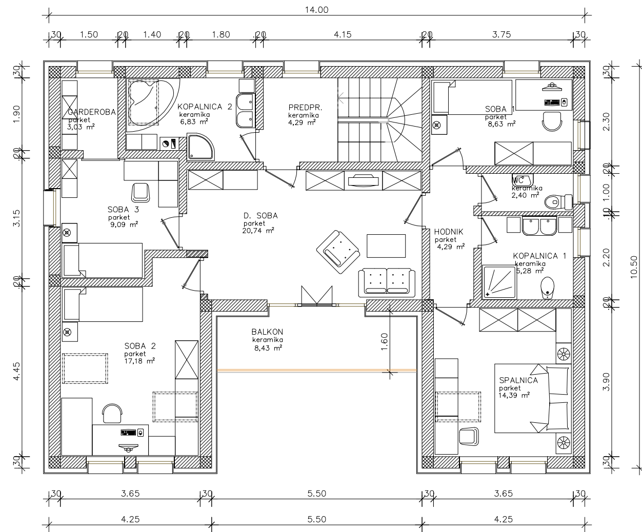
TLORIS MANSARDE
