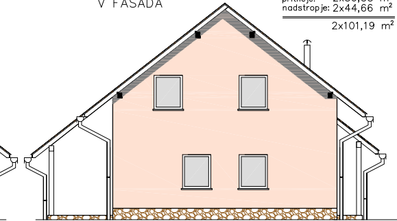
V FASADA
