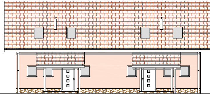
S FASADA
