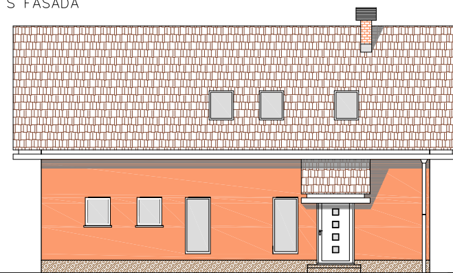
S FASADA
