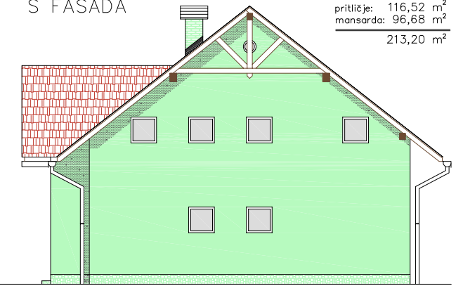
S FASADA
