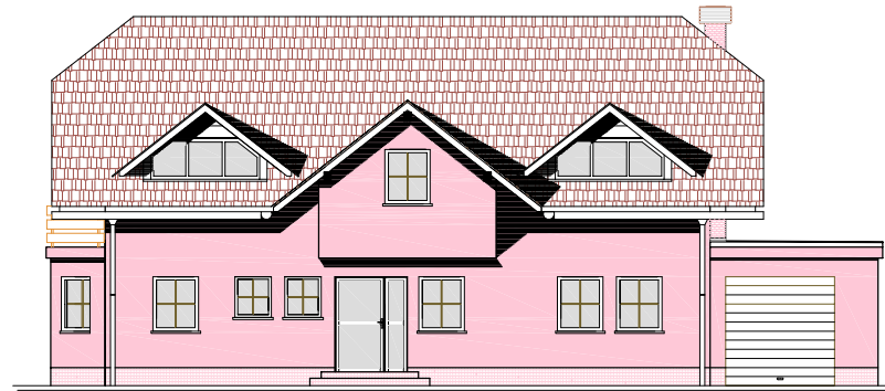
V FASADA
