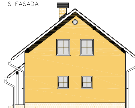
S FASADA
