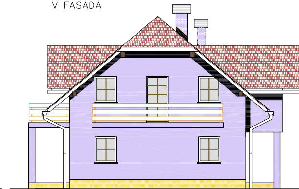
V FASADA
